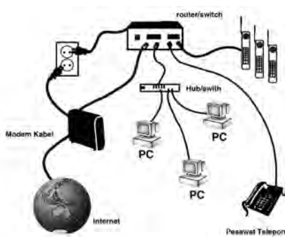
Gambar 2.2. Skema koneksi internet menggunakan saluran TV Kabel
