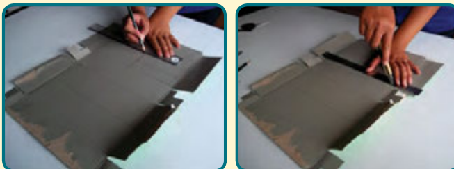
Sumber: Dok. Kemendikbud Gambar 1.54. Pembuatan pola pada kotak bekas
