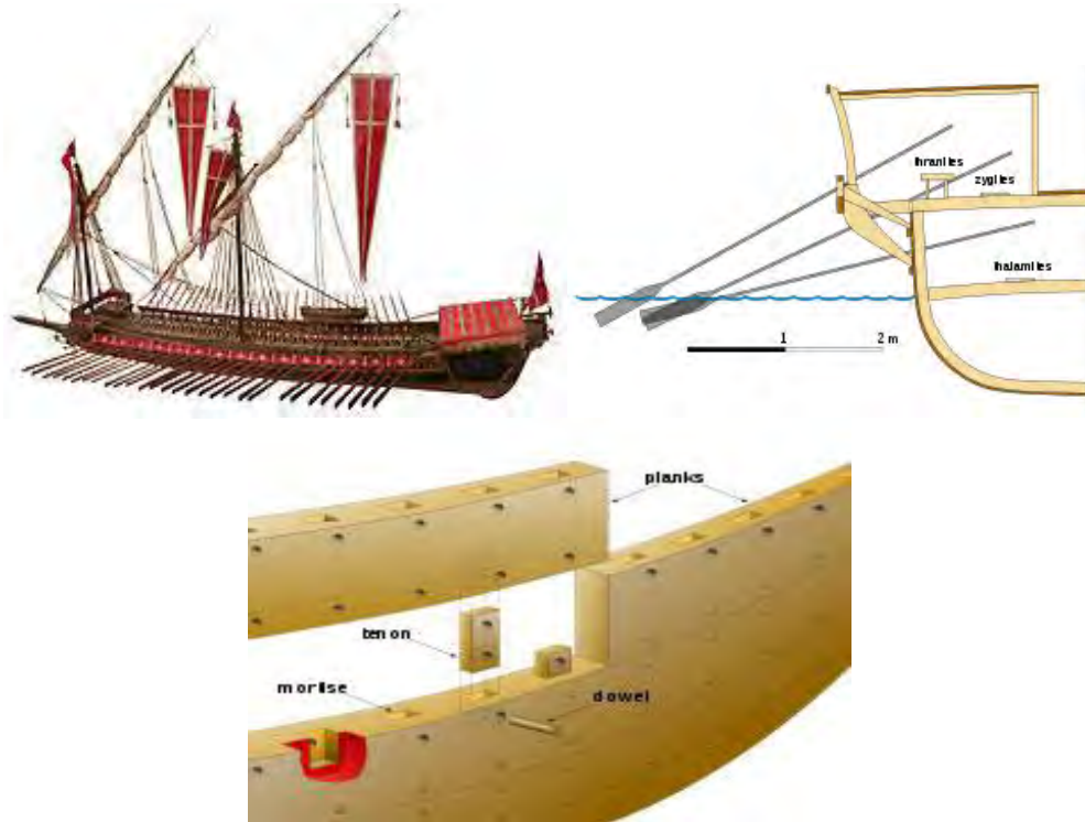
Gambar 11. Kapal layar dayung jenis galley. Sistem penyusunan dan penempatan dayung (kana)
