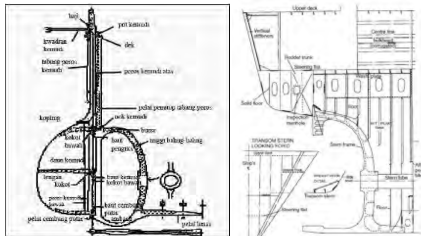
Gambar 53. Beberapa contoh konstruksi daun kemudi
