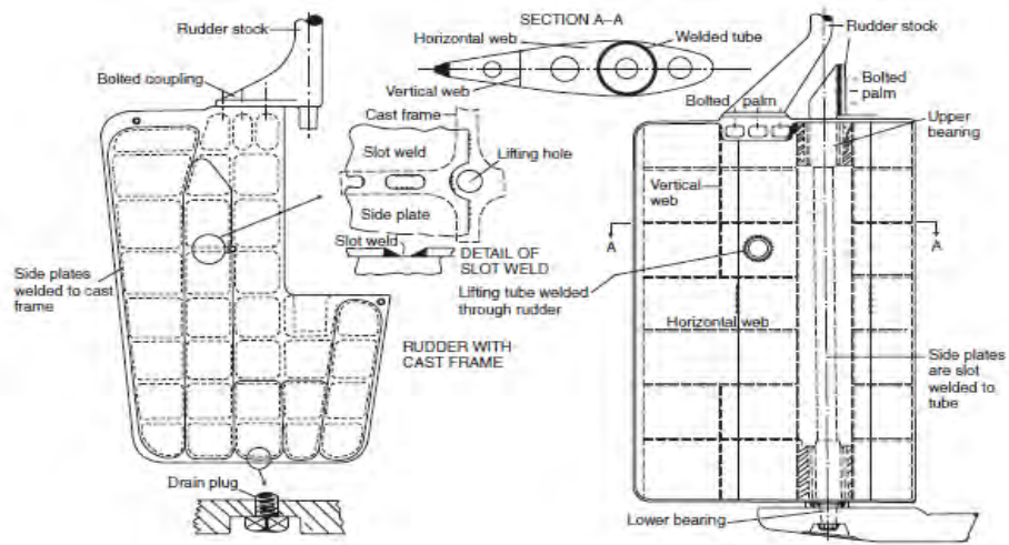
Gambar 51. Konstruksi kemudi
