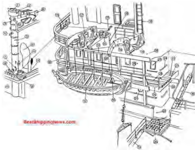
Gambar 84. Alat bantu di deck sekoci
