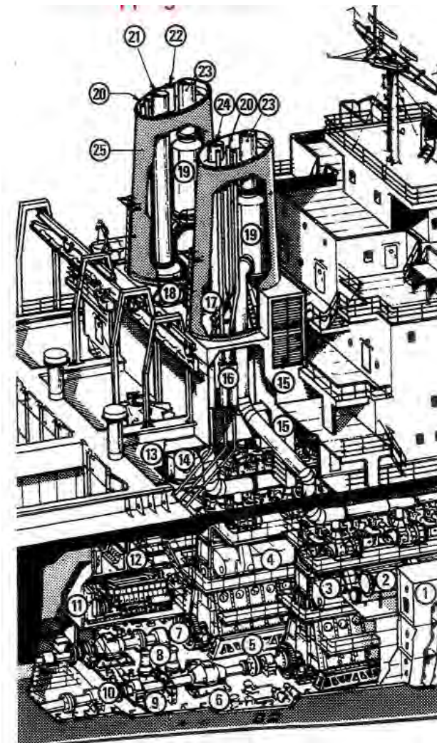
Gambar 49. Ruang mesin
