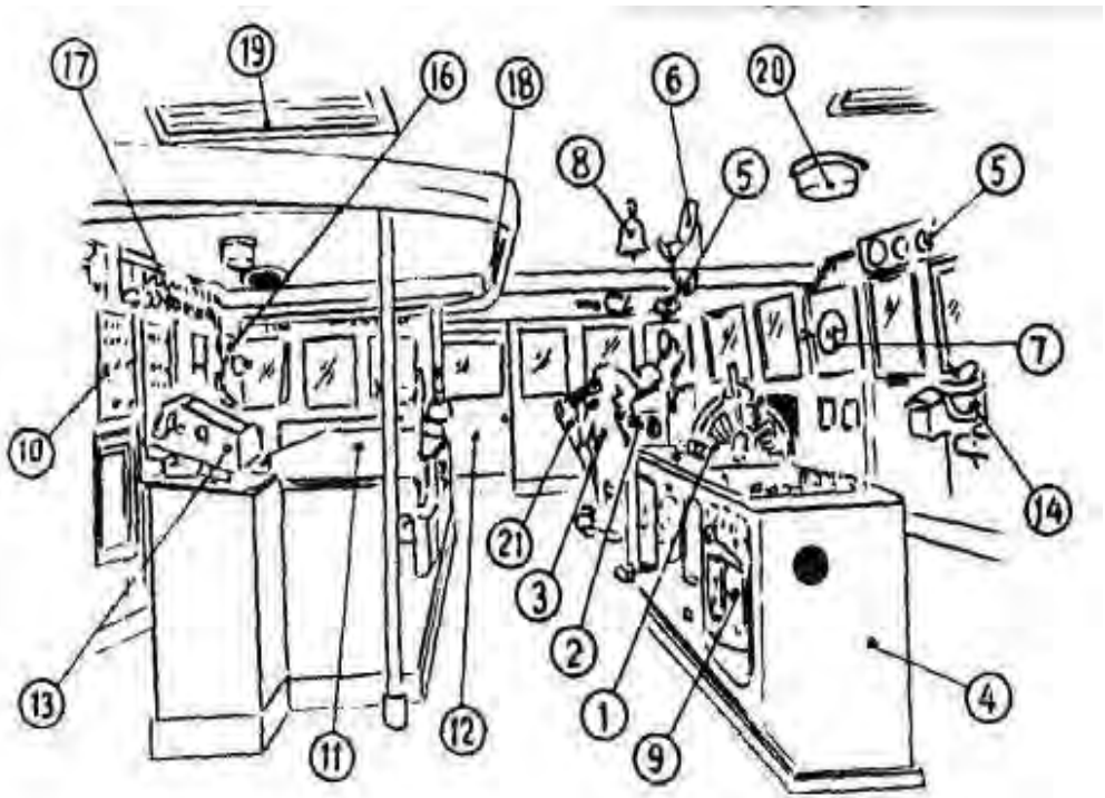
Gambar 42. Ruang anjungan
