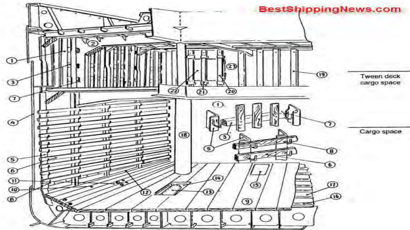
Gambar 47. Ruang barang
