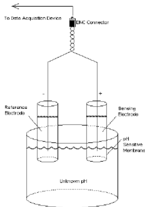
Gambar 31. Elektroda Potensiometrik
