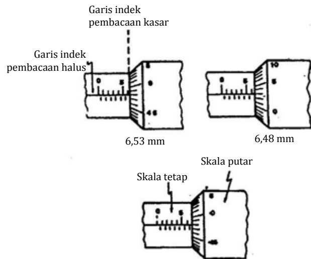
Gambar 19. Pembacaan skala pengukuran dengan mikrometer
