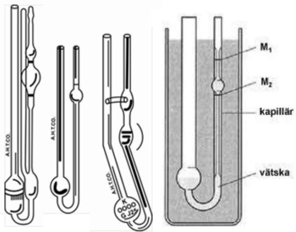
Gambar 23. Viskosimeter Oswald
