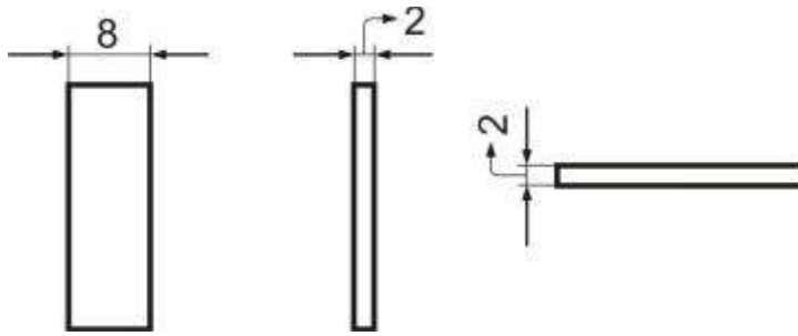
Gambar 2.18. Penulisan garis dan angka ukuran untuk ukuran yang pendek
