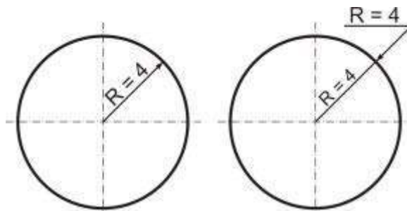
Gambar 2.19. Penulisan garis ukuran jari-jari lingkaran
