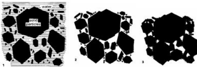
Gambar 6.14. Porositas tanah liat setelah proses pembakaran. (sumber: Frank Hammer)
