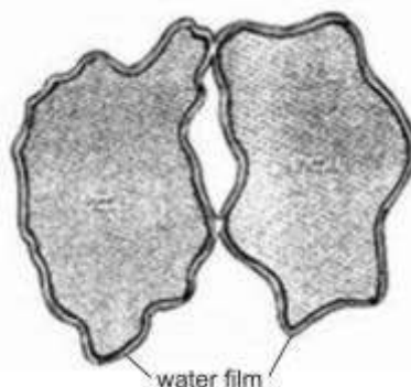
Gambar 6.5. Dua partikel kwarsa dengan lapisan air. (sumber: F.H. Norton)
