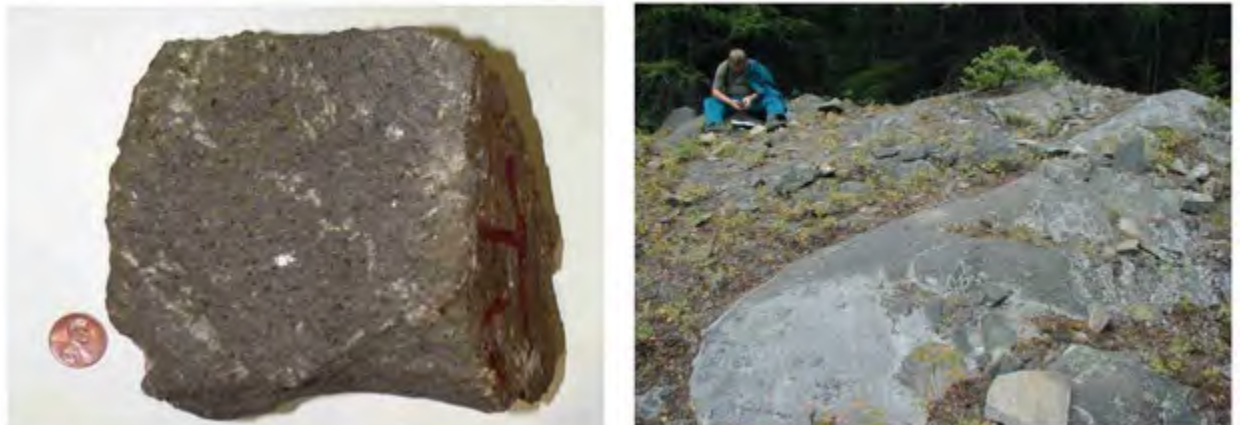
Gambar : Batuan beku vulkanik, Jenis batuan beku intermediate, nama : batu Andesite
