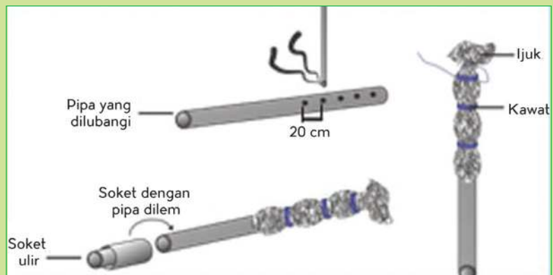
Gambar 2.9. Pipa penyaring
