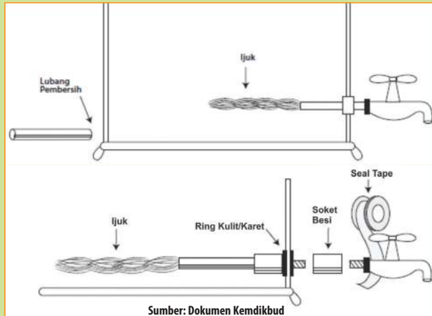
Gambar 2.19 Pipa penyangkang
