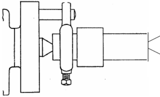
Gambar 2.28: Pemasangan benda kerja, bubut eksentrik
