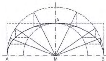
KONSTRUKSI ELLIPS 3
