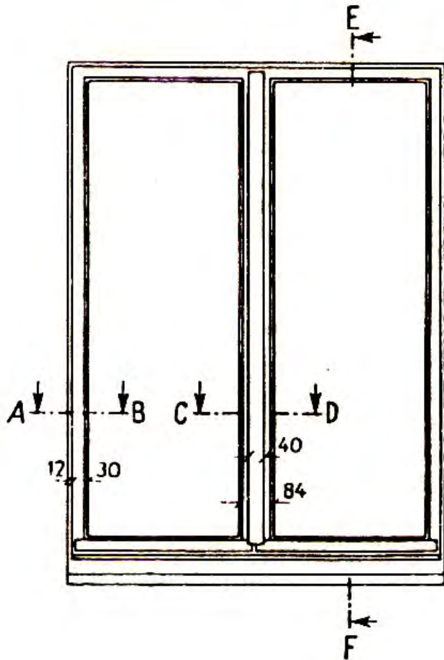
Gambar 4. 6 Kusen Jendela doble
