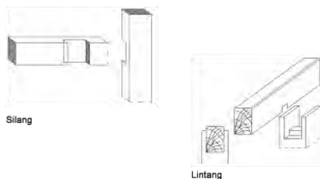
Gambar 4. 23 Hubungan Kayu silang
