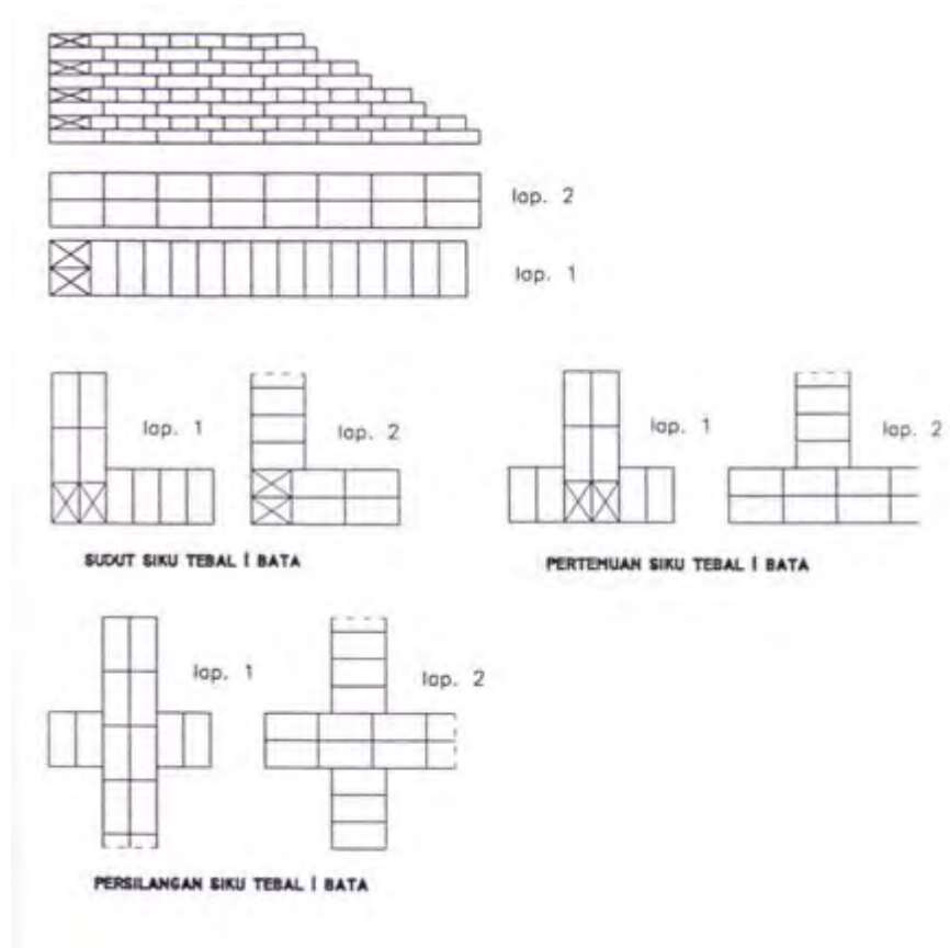
Gambar 3. 5 Ikatan Tegak
