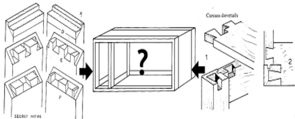
Contoh Pekerjaan Konstruksi "Carcase"
