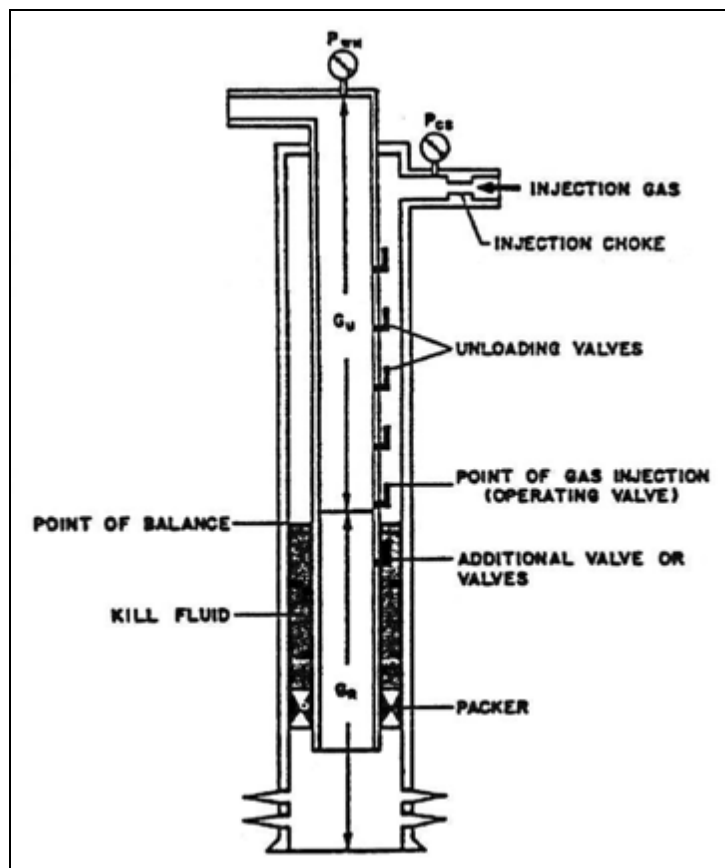
Gambar 8.6. Operasi Gas-Lift Aliran Kontinyu
