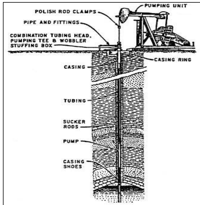
Gambar 8.8. Sistem Pemompaan Beam
