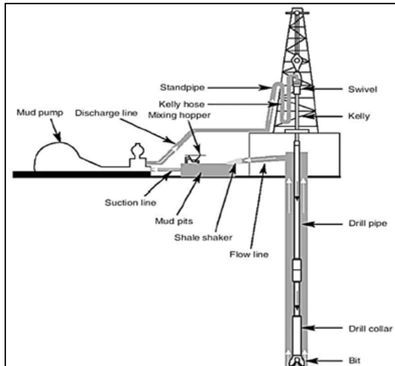
Gambar 4.31. Sistem Sirkulasi
