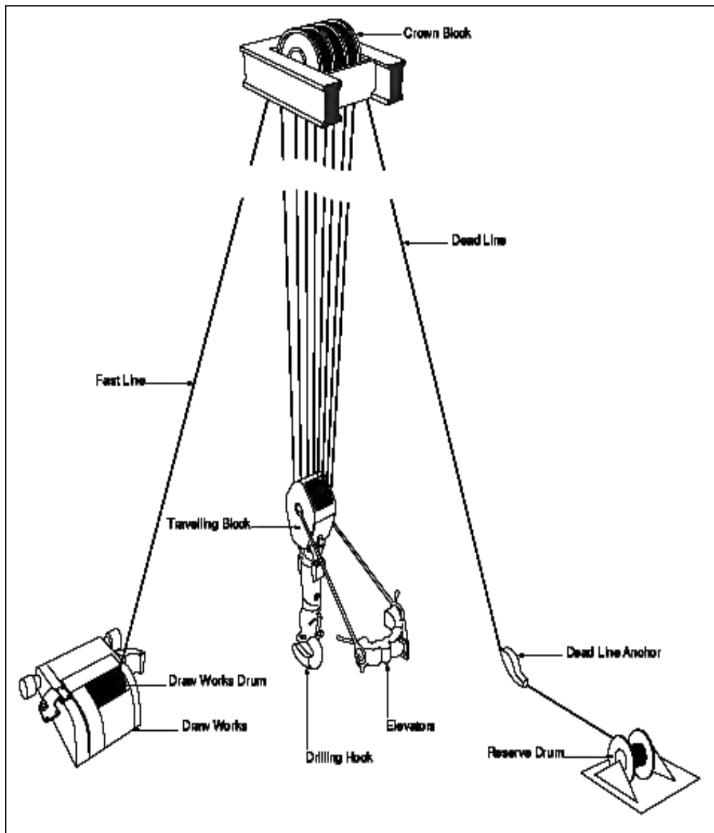
Gambar 4.2. Sistem Angkat ( hoisting system )
