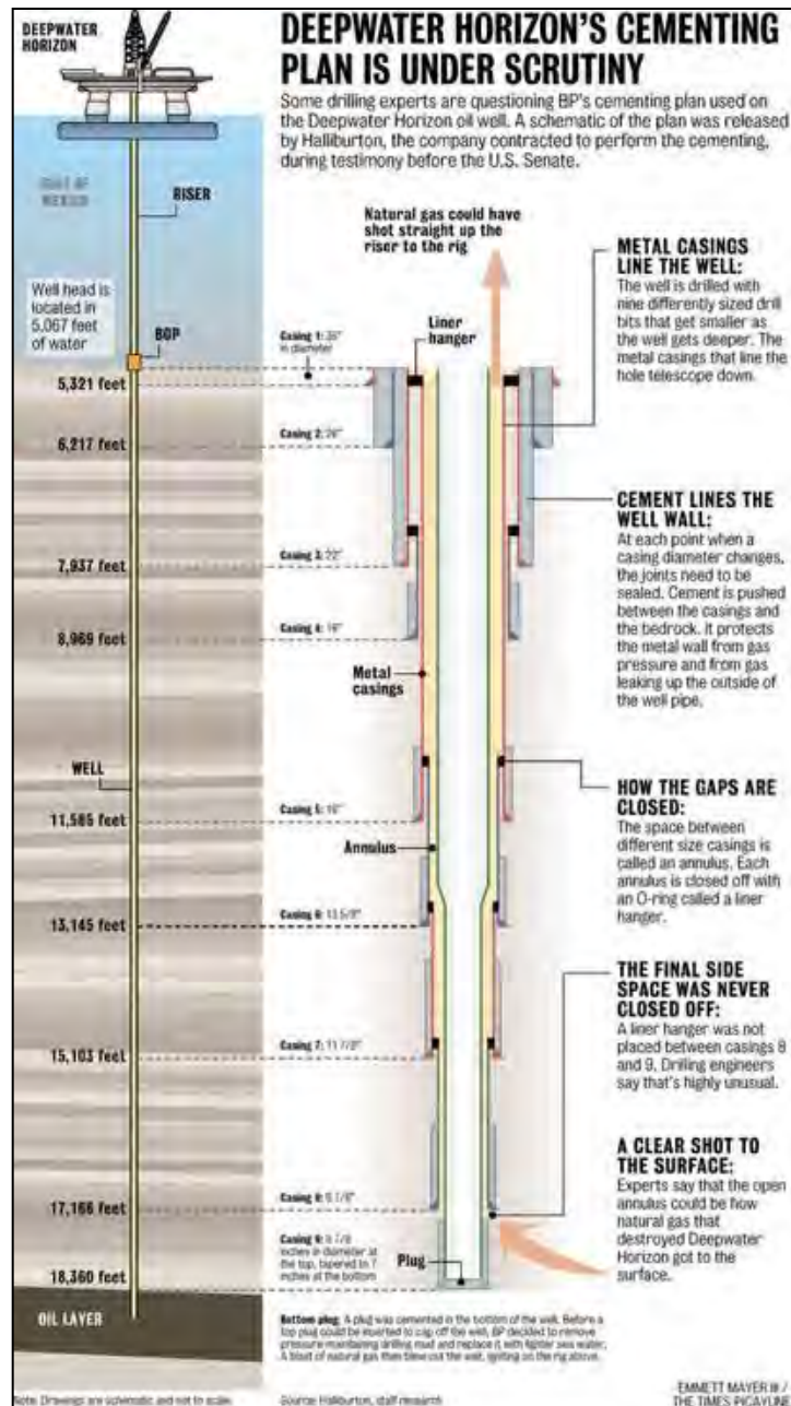
Gambar 5.1. Contoh Konstruksi Sumur Pengeboran
