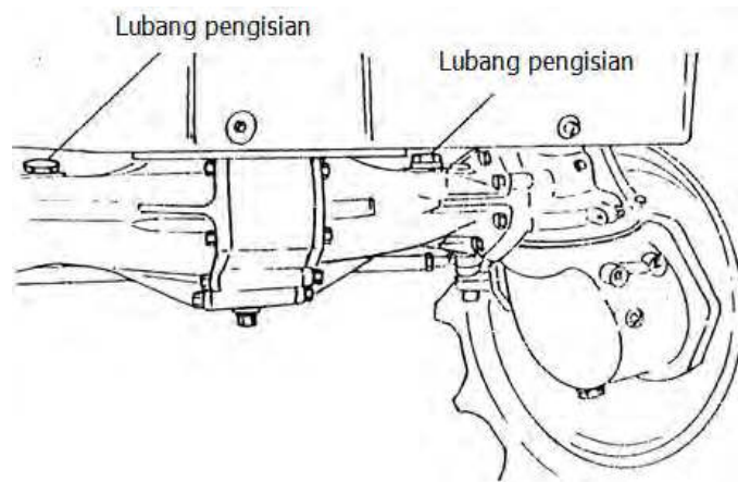
Gambar 46. Lubang pengisian oli gardan depan
