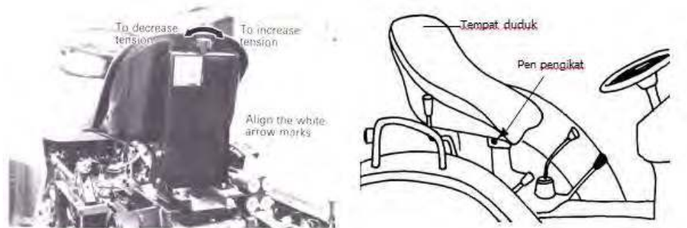
Gambar 32. Pengatur tempat duduk
