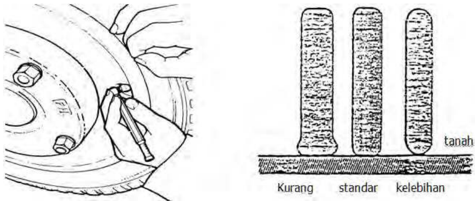
Gambar 47. Cara mengukur tekanan dan kenampakan kondisi ban
