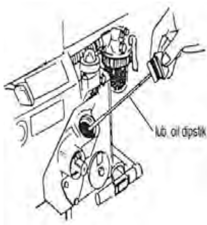
Memeriksa oli mesin
