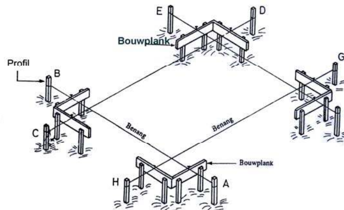
Gambar III-9, Pekerjaan Uitzet dan Bouwplank
