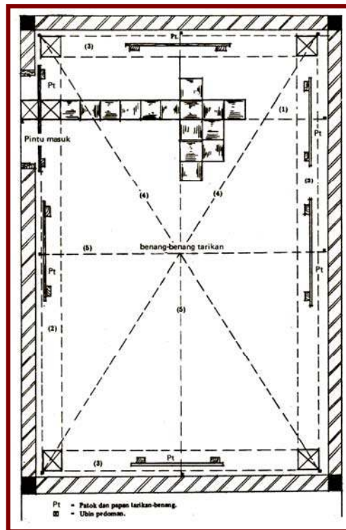
Gambar VI-1, Ketentuan Umum Pemasangan Ubin Lantai
