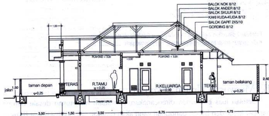
Gambar I-8, Gambar Potongan Memanjang
