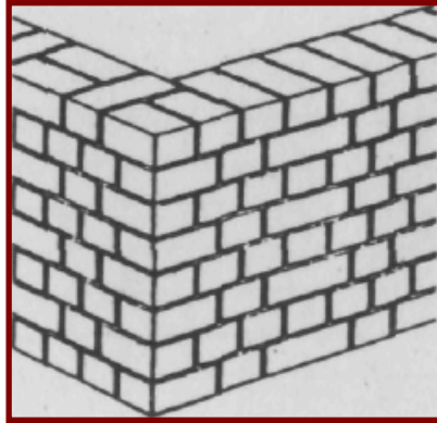
Gambar IV-27. aturan batu Belanda
