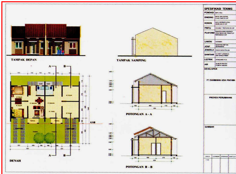
Gambar I-13, Gambar Rencana
