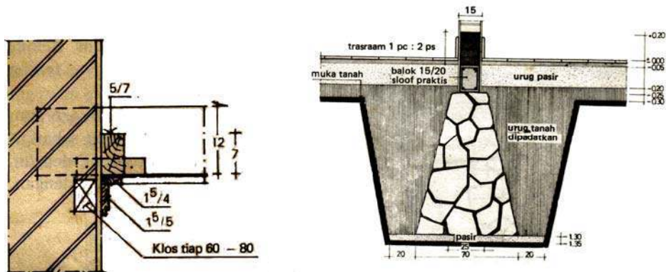
Gambar I-5, Gambar Kerja Detail Hubungan Plafon dan Bentuk Pondasi
