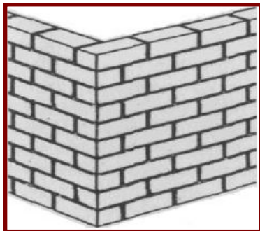
Gambar IV-23. Aturan batu memanjang (1/2 batu) dengan tebal dinding 11 cm atau 11,5 cm
