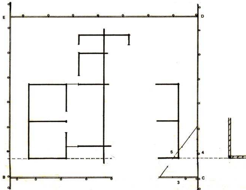
Gambar III-4, Pemasangan Bouwplank di Sekeliling Bangunan
