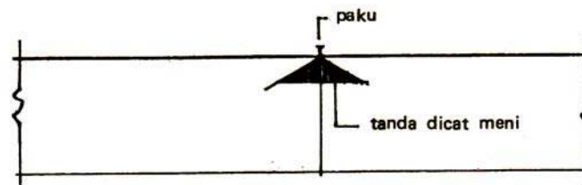
Gambar III-6, Pemberian Tanda pada Bouwplank
