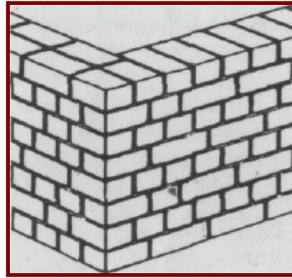
Gambar IV-26. aturan batu menyilang
