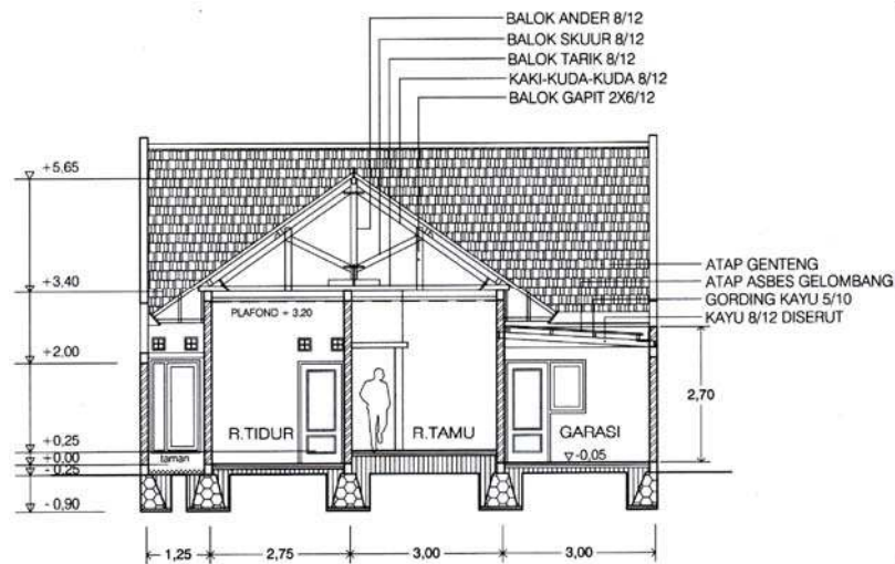
Gambar I-7, Gambar Potongan Melintang
