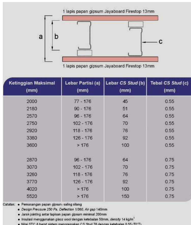
Gambar IV-12. Potongan/tampak atas dan spesifikasi produk dinding partisi
