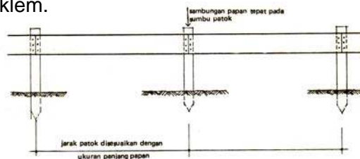
Gambar III-7, Sambungan Papan pada Patok
