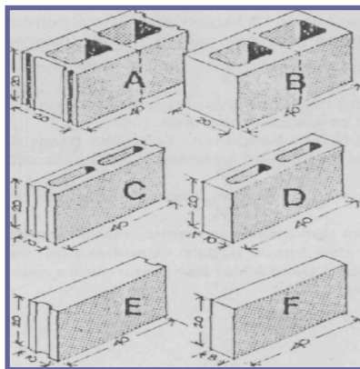
Gambar IV-15. Beberapa macam bentuk batako
