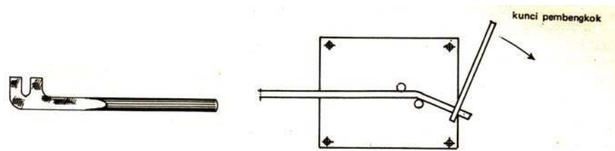
Gambar VIII-2, Kunci Pembengkok dan Cara Membengkok Besi
