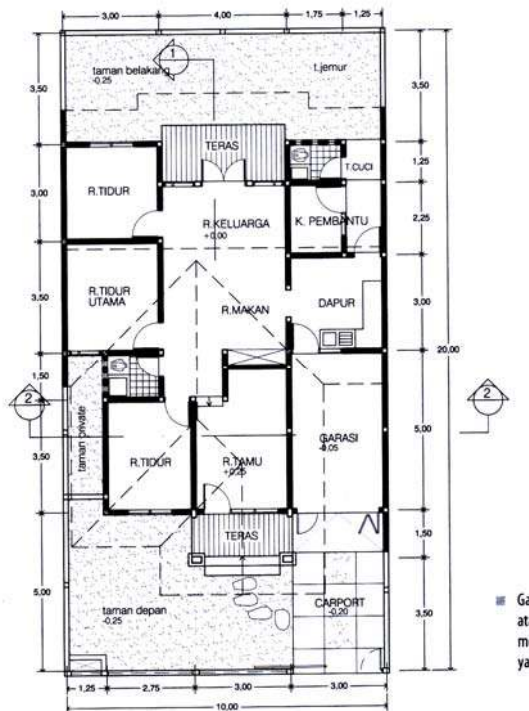
Gambar I-6, Gambar Denah
