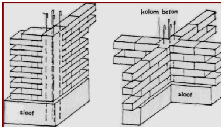
Gambar IV-30. Cara pemasangan batu bata dengan kolom beton
