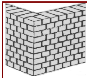
Gambar IV-24. aturan batu melintang
