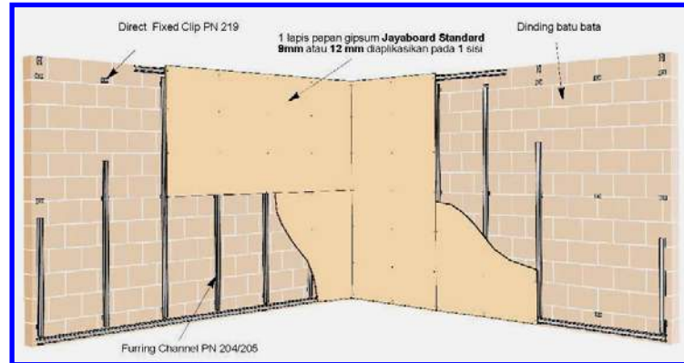
Gambar VI-12. Sistem pelapis dinding batu ini menggunakan 1 lapis papan gipsium. Furring Channel dan Direct Fixed Clip, diaplikasikan pada 1 sisi. Rongga yang terdapat di antara papan gipsium dan dinding batu dapat difungsikan untuk instalasi ME (mekanikal-elektrikal) atau insulasi (jika diperlukan).
