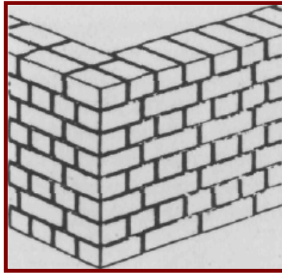
Gambar IV-25. Aturan batu memanjang-melintang bersilang (staand)
