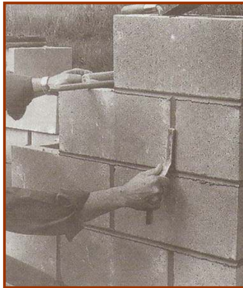
Gambar IV-16, Mesin Cetak Batako dan pemasangan batako
