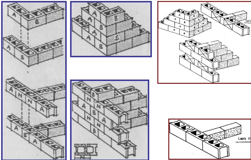
Gambar IV-18, Beberapa aturan pemasangan batako
