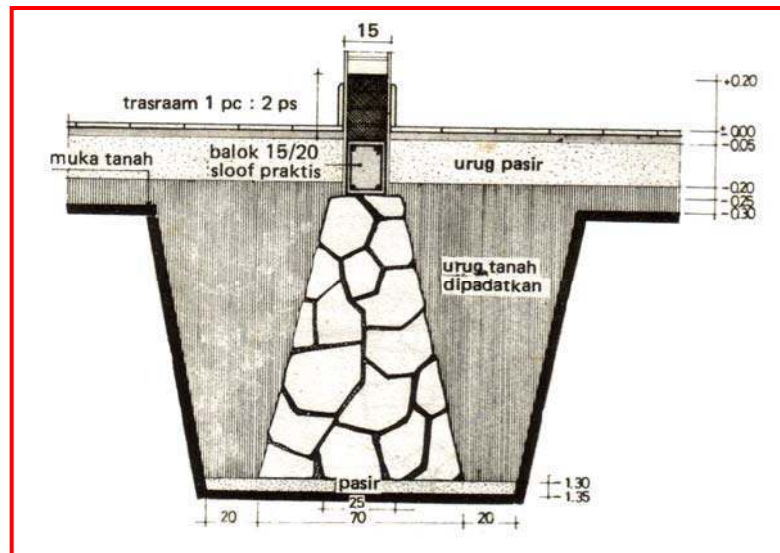
Gambar IV-3, Konstruksi Pondasi Batu Kali
