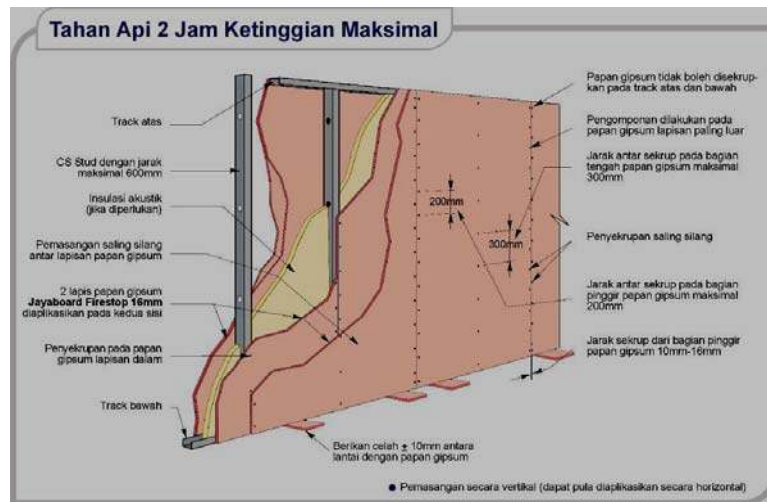
Gambar IV-13. Sistem Partisi Tahan Api 2 Jam Ketinggian Optimal, menggunakan 2 lapis papan gipsium 16mm yang diaplikasikan pada kedua sisi dan rangka BMS dengan tebal (TCT) min 0.55mm
