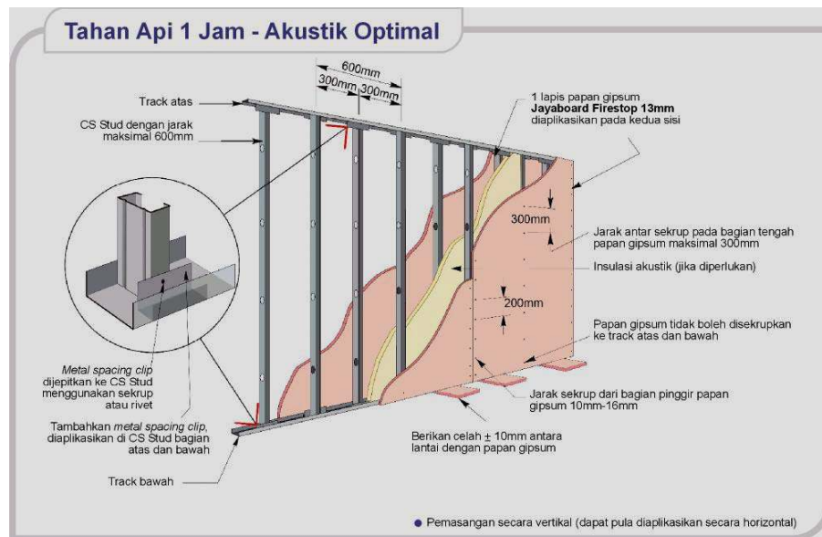
Gambar IV-11. Sistem Partisi Tahan Api 1 Jam - Akustik Optimal, menggunakan 1 lapis papan gipsium 13mm yang diaplikasikan pada kedua sisi dan rangka BMS yang diaplikasikan saling-silang ( staggered ) dengan ketebalan (TCT) minimal 0.55mm
