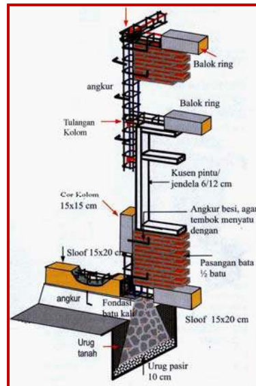
Gambar I-4, Gambar Kerja Hubungan Sloof, Kolom, dan Ring balok
