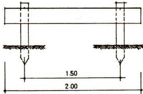
Gambar III-5, Pemasangan Bouwplank di Sudut/Pertemuan Dinding
