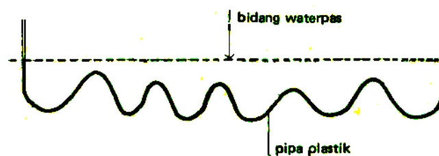
Gambar III-1, Membuat Bidang Waterpass dengan Selang Plastik
