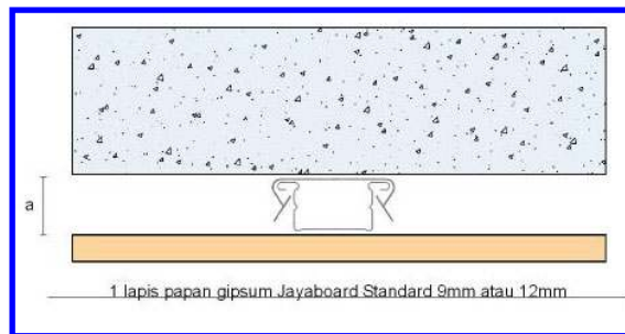
Gambar VI-13. Potongan samping pelapis dinding
