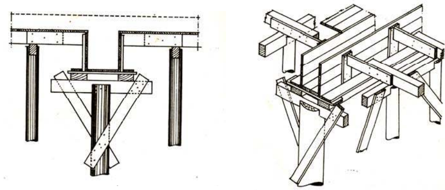
Gambar VIII-1, Acuan dan Perancah
