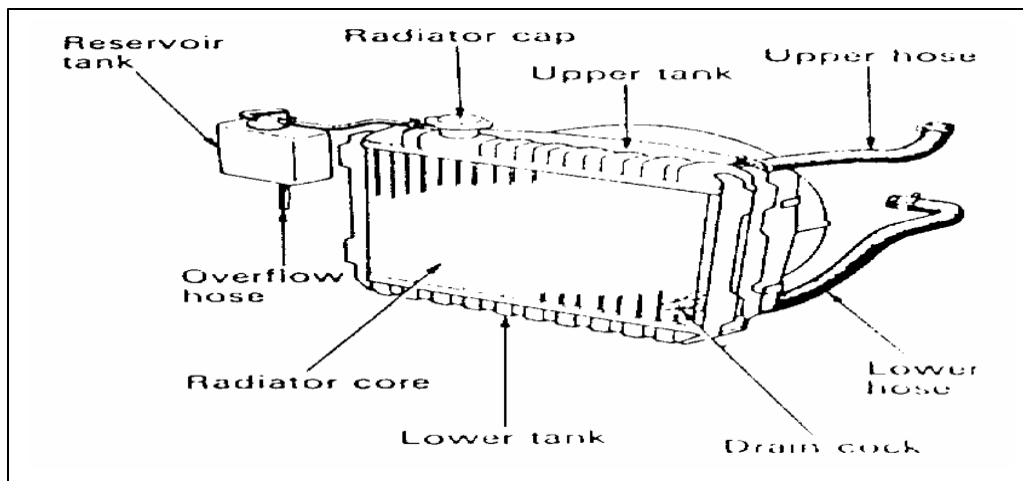
Gambar 4.20. Pembagian Radiator
