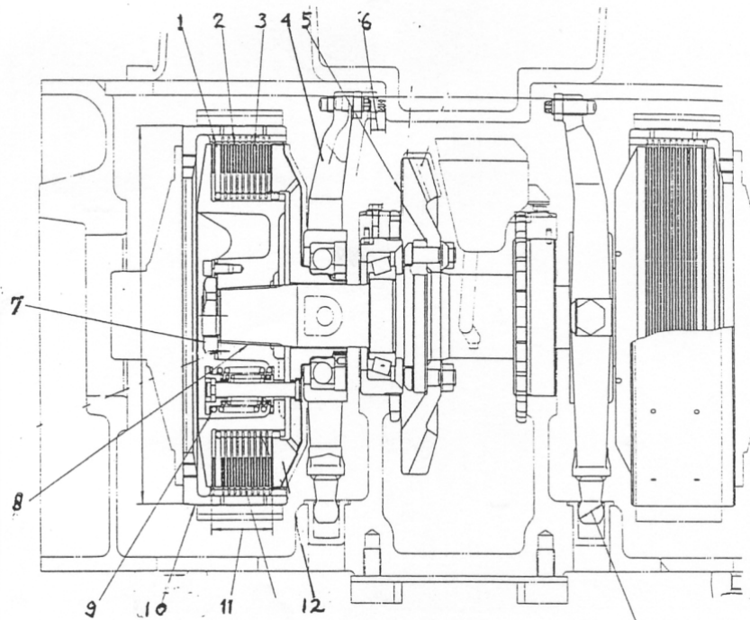
Gambar 4.118 Konstruksi Steering Clutch .
