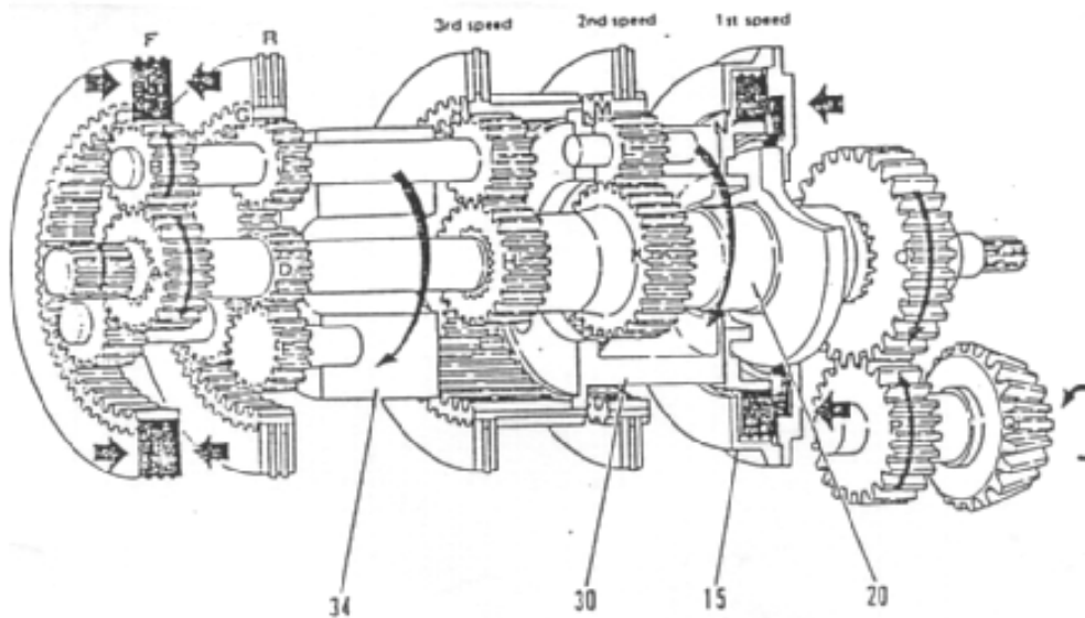
Gambar 4.207 Maju Kecepatan 1
