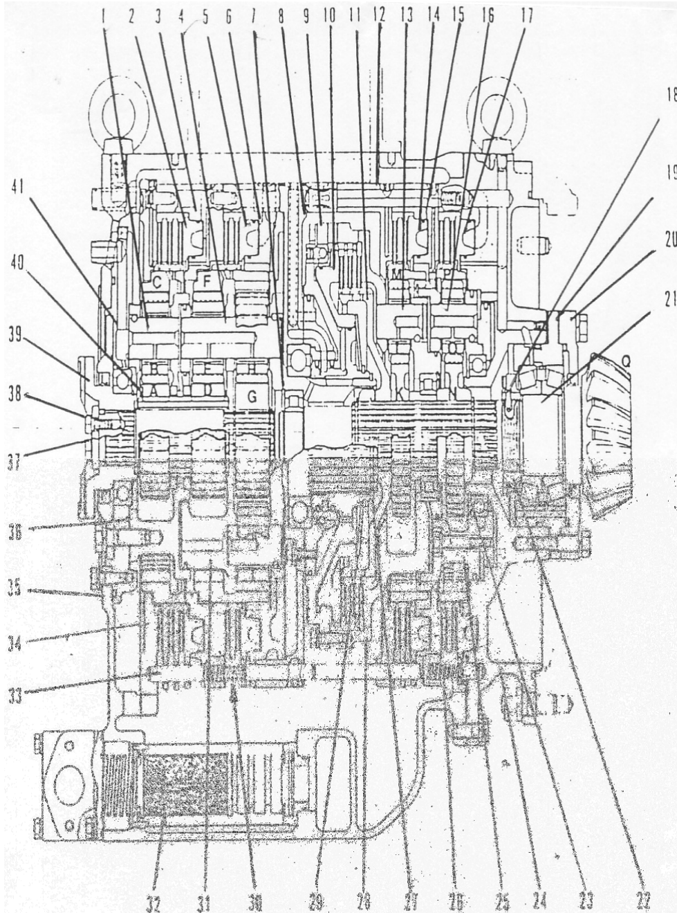
Gambar 4.195. Konstruksi Torqflow Transmission
