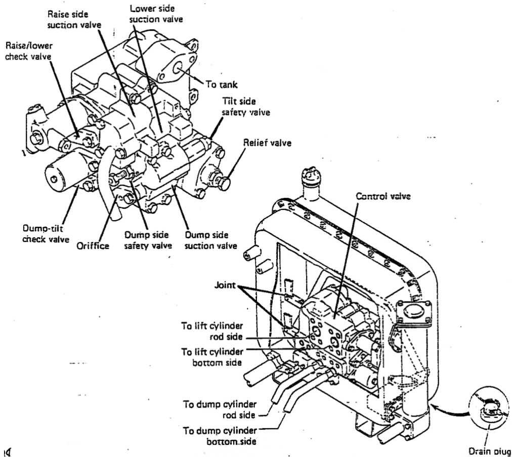
Gambar 4.106. Contoh bentuk control valve pada dozer shovel
