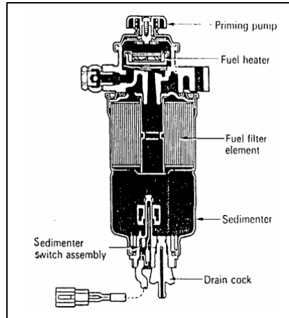
Gambar 4.40. Saringan Bahan Bakar dan Water Sedimenter
