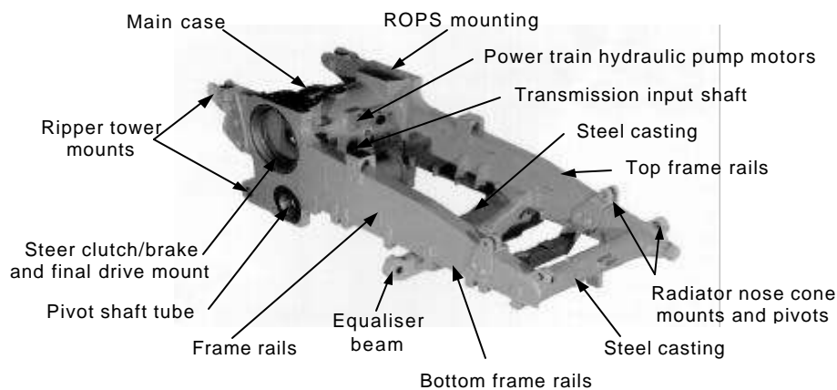
Gambar 4.151 Frame traktor jenis tract
