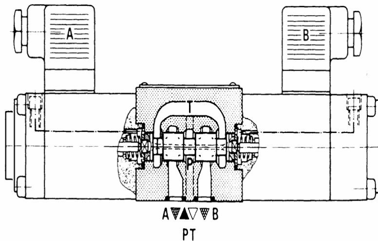
Gambar 4.88 Solenoid ganda yang dioperasikan dengan katup tiga posisi.
