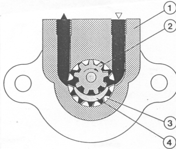
Gambar 4.64 Pompa roda gigi dalam
