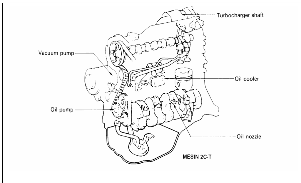
Gambar 4.31. Skema Aliran Pelumasan
