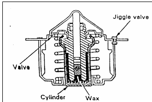
Gambar 4.26. Thermostat Dengan Wax
