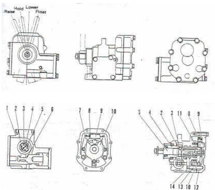
Gambar 4.135 Konstruksi blade lift servo valve
