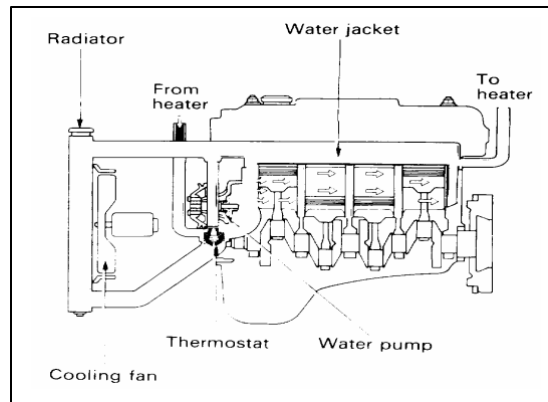
Gambar 4.19. Proses Pendinginan Saat Mesin Panas
