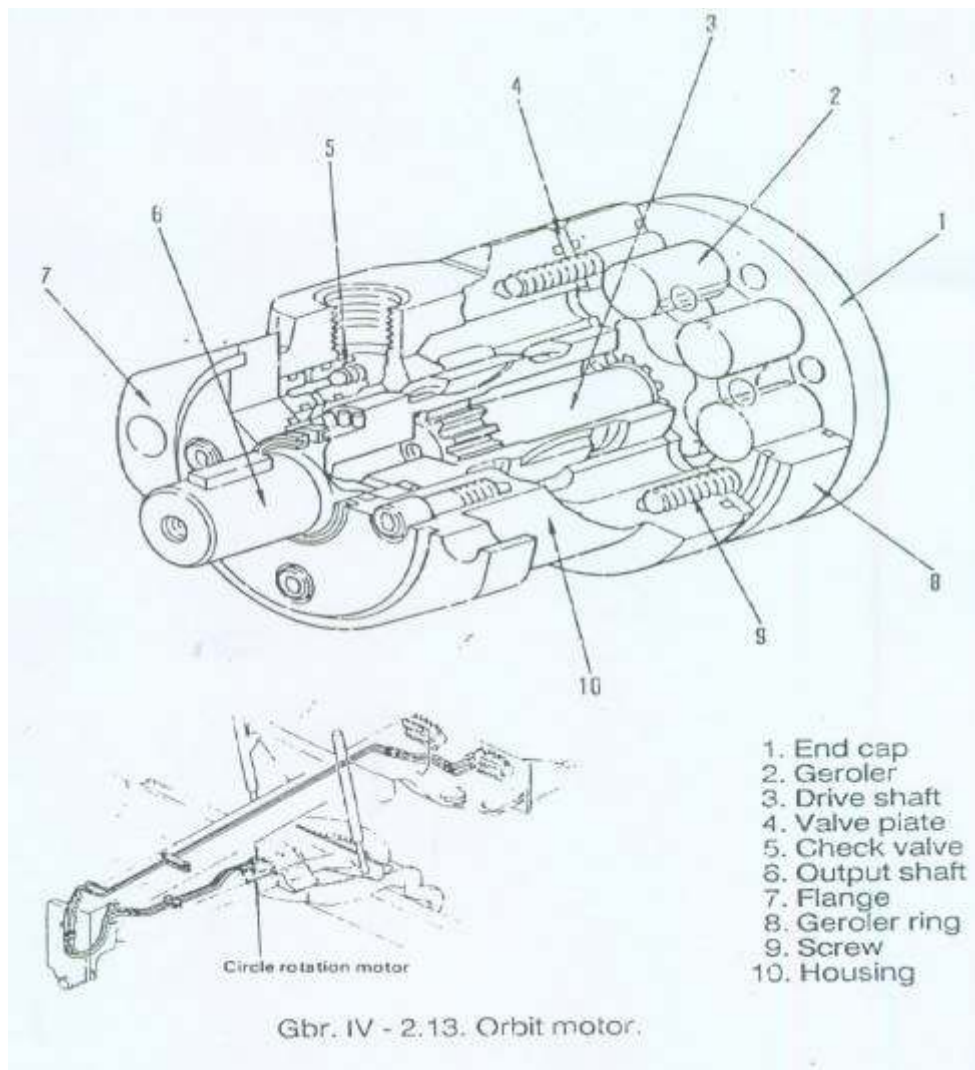
Gambar 4.162 Konstruksi Orbit Motor
