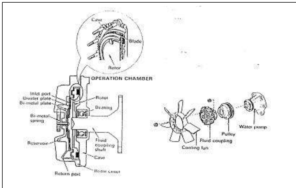
Gambar 4.28. Kipas Radiator dan Kopling Fluida ( fluid clutch )
