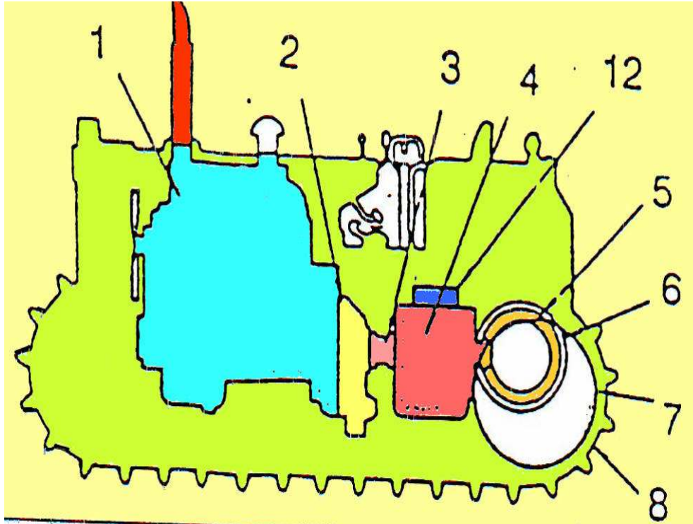
Gambar 5.20 Nama Bagian Bulldozer
