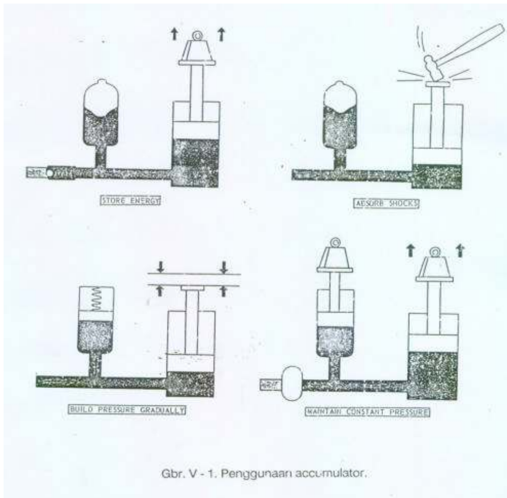
Gambar 4.166 Penggunaan akumulator
