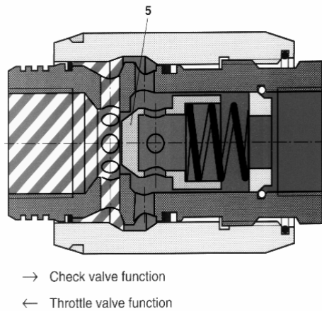
Gambar 4.98 Katup check dan throttle
