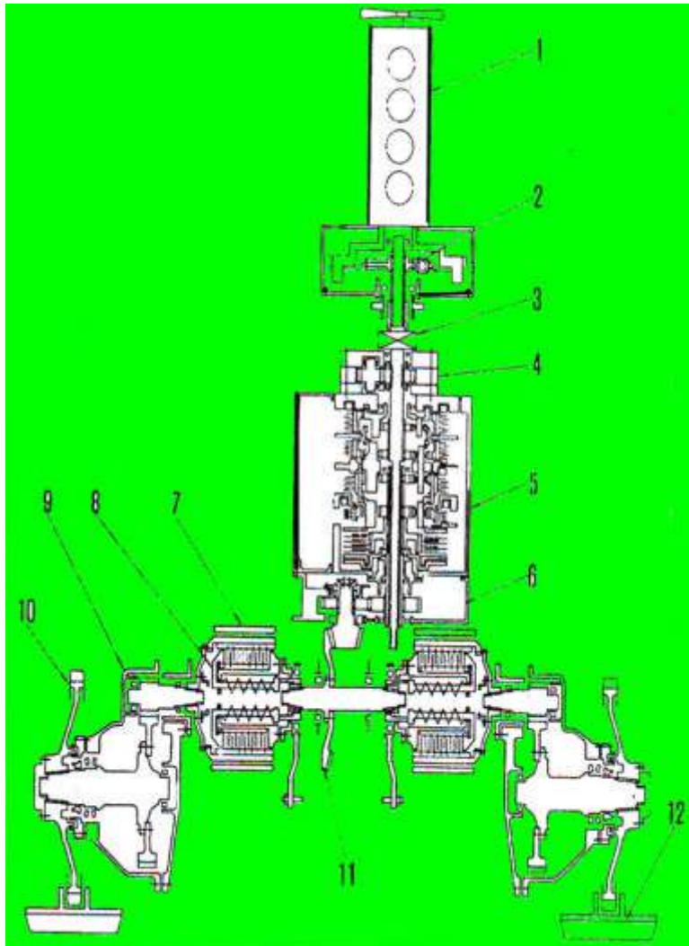
Gambar 23 Buldozer dengan hydrosift system.
