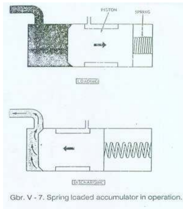
Gambar 4.170 Cara kerja akumulator pegas
