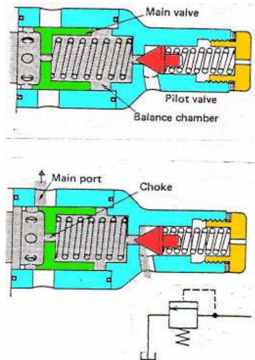
Gambar. 4.109 Simbul dan prinsip kerja tipe pilot
