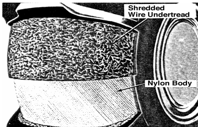
Gambar 4.145 Jalinan kawat pencegah sobekan (SWB)
