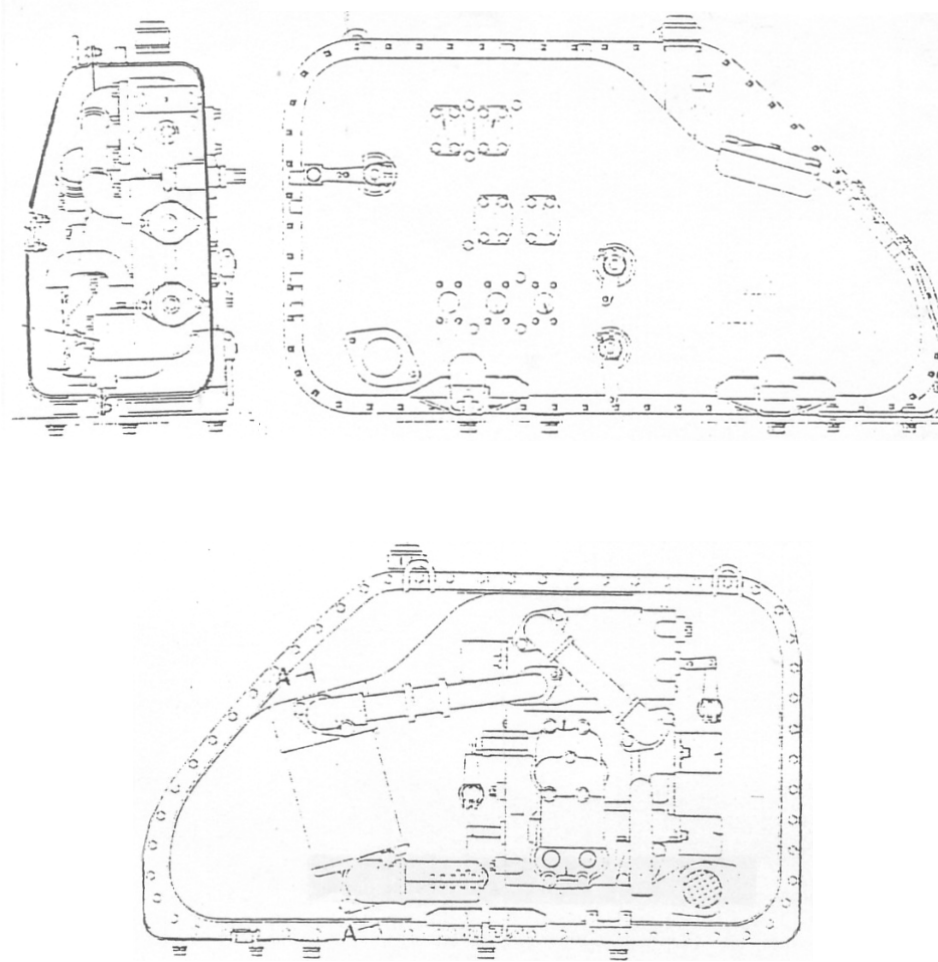
Gambar 4.51. Konstruksi Tangki Hidrolik
