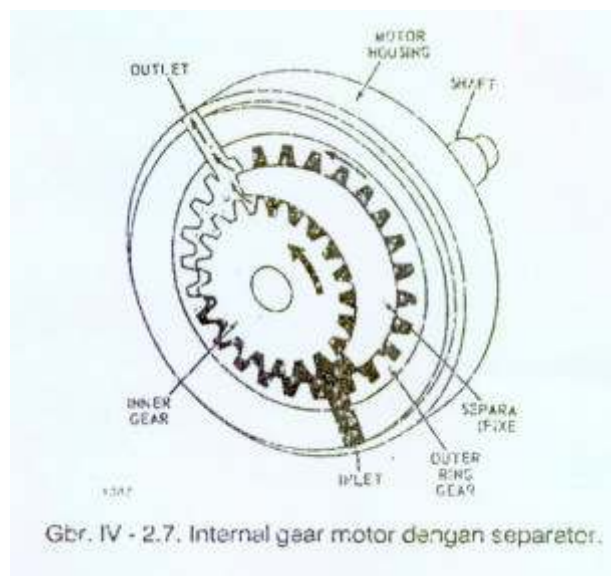
Gambar 4.157 Internal gear motor dengan separator
