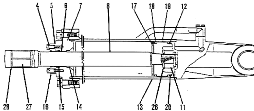
Gambar 4.138 Contoh silinder hidrolik Blade Tilt Cyl untuk D85
