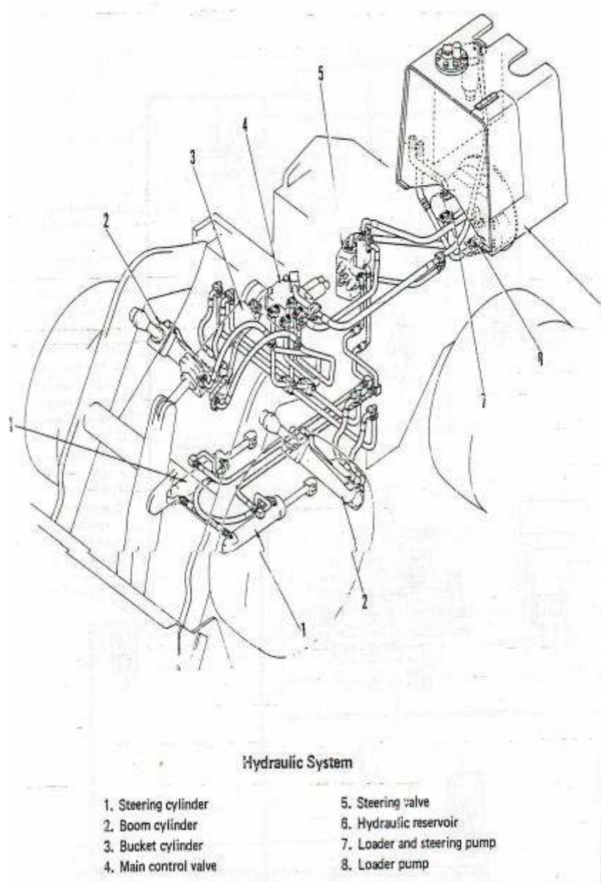
Gambar 4.122 (a) Konstruksi kendaraan Wheel Loader
