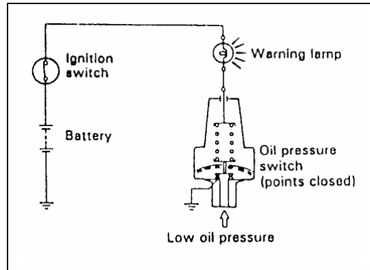
Gambar 4.35. Switch Oli Memassakan Lampu
