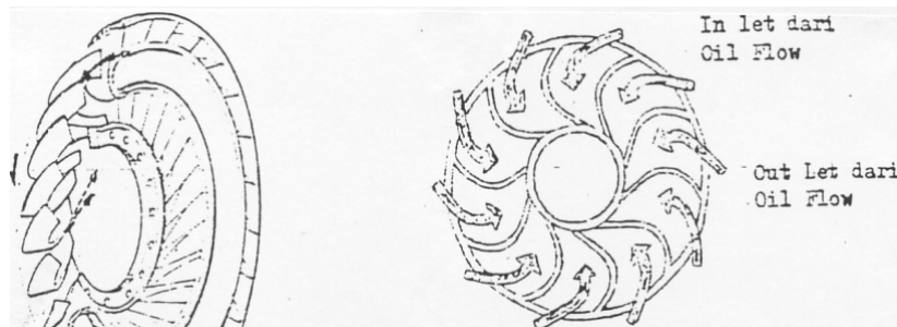
Gambar 4.173 Turbin pada Torque Converter
