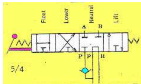
Gambar 4.127 Simbul katup pengontrol arah aliran (5/4)
