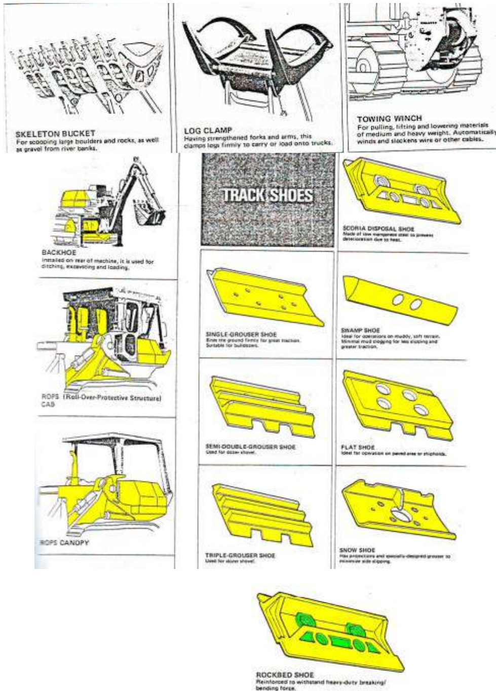
Gambar 5.27 Perlengkapan Doser Shovel (2)
