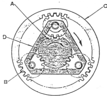
Gambar 4.199 Planetary Gear dengan Ring Gear ditahan A ditahan
