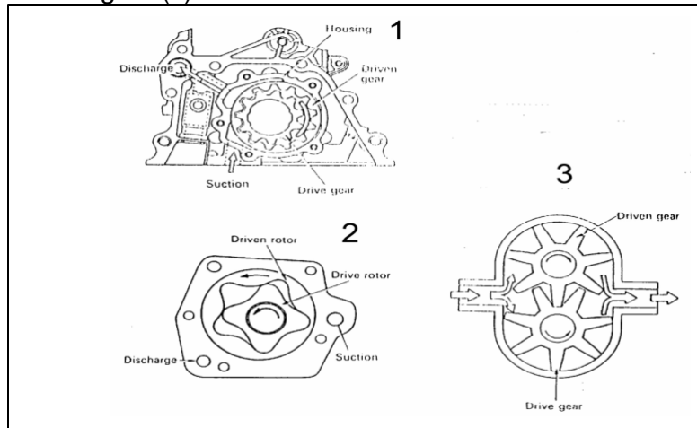
Gambar 4.32. Macam-macam Pompa Oli
