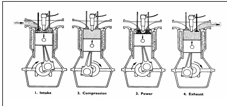
Gambar 4.15 Siklus Pembakaran Motor Diesel 4 Tak
