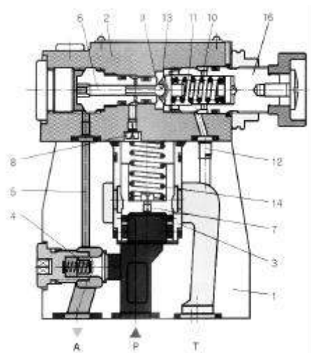
Gambar 4.100 Katup shut-off dengan pemandu tekanan
