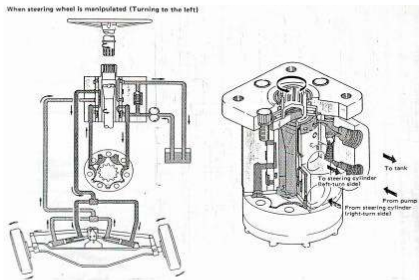
Gambar 4.132 (d) Prinsip kerja orbitrol valve sebagai hand pump
