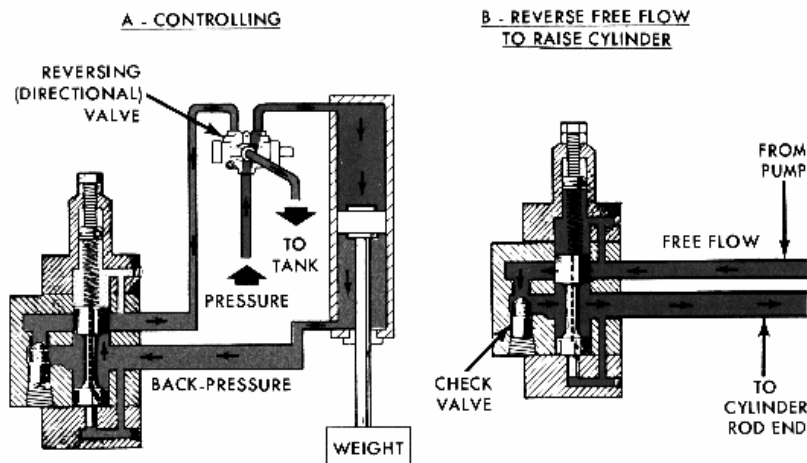
Gambar 4.102 Katup penyeimbang
