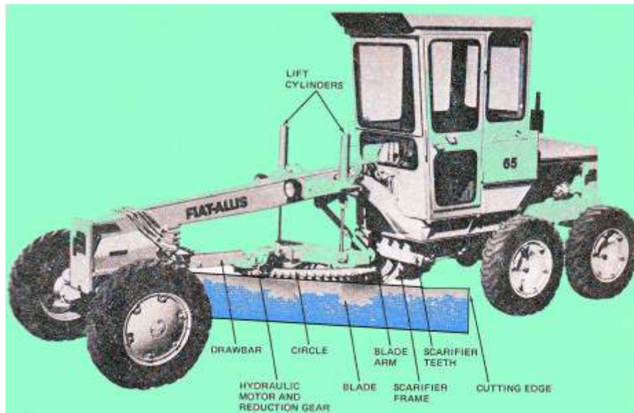
Gambar 5.16 Nama komponen Motor Grader
