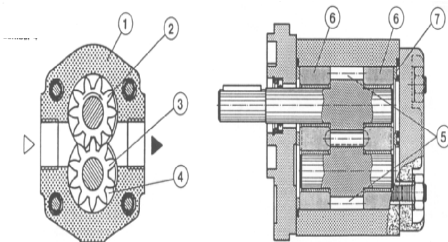
Gambar 4.65 Pompa roda gigi dengan roda gigi luar
