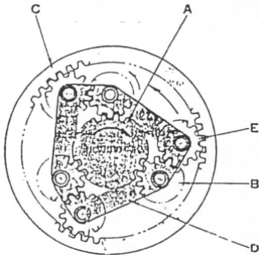
Gambar 4.201 Cara kerja Double Pinion Type
