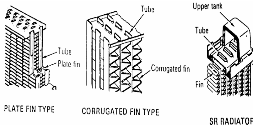
Gambar 4.21. Tipe- tipe Radiator
