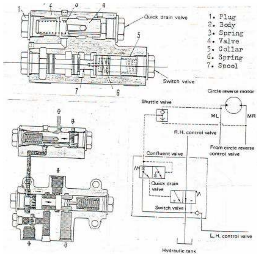
Gambar 4.137 Konstruksi, symbol dan prinsip kerja confluent valve
