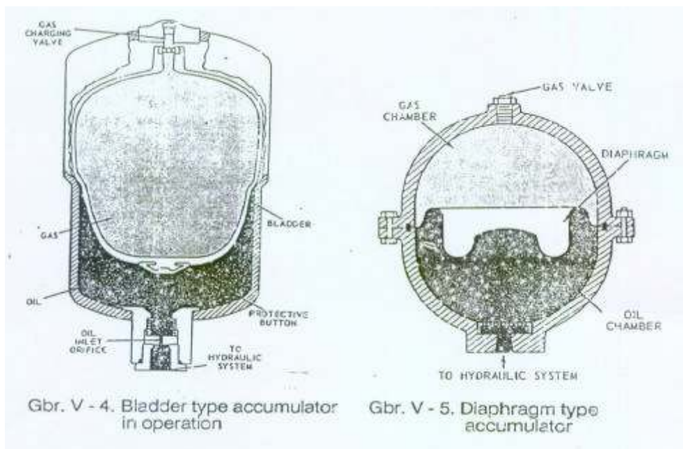
Gambar 4.168 Akumulator type bladder dan diaphragma
