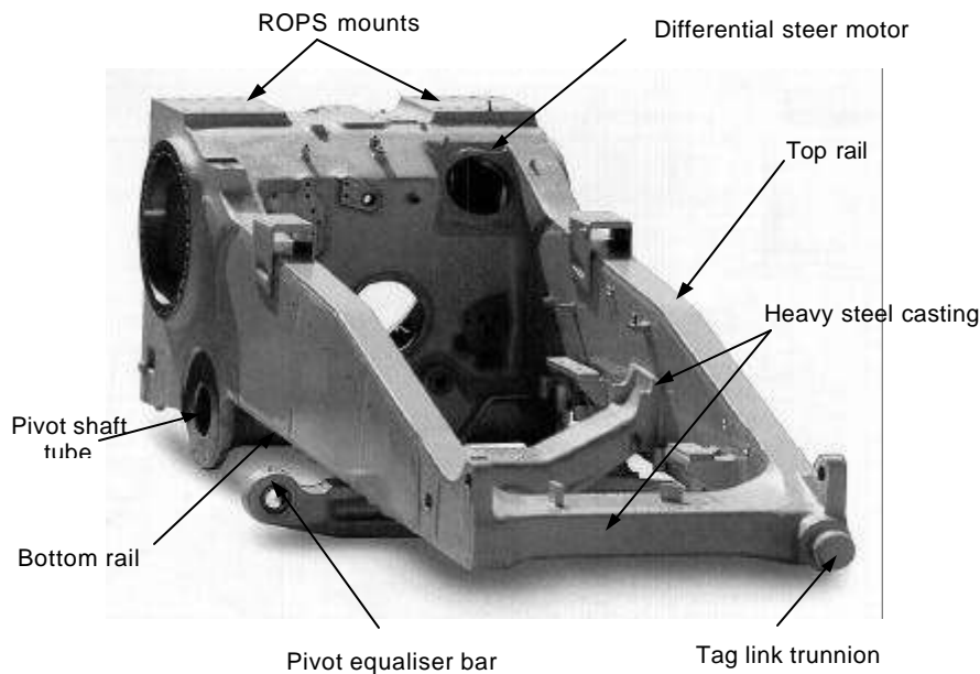
Gambar 4.152 Frame traktor jenis track
