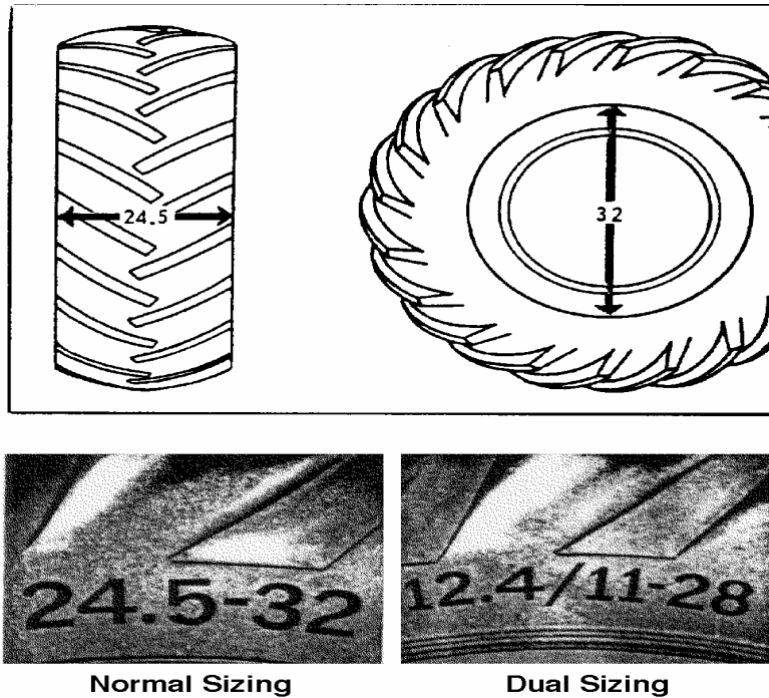
Gambar 4.149 Jenis tanda ukuran pada ban
