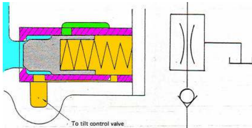
Gambar 4.115 Flow reducing valve & simbol (belum bekerja)
