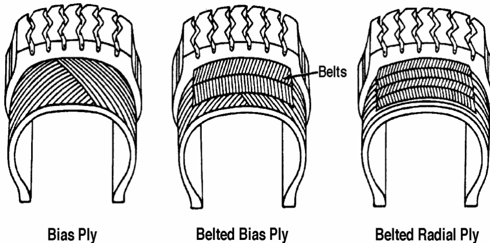
Gambar 4.144 Bias ply pada ban
