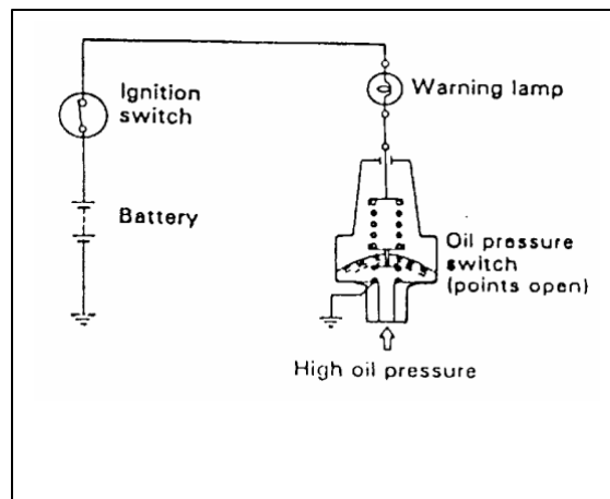
Gambar 4.36. Switch Oli Memutuskan Lampu Dengan Massa
