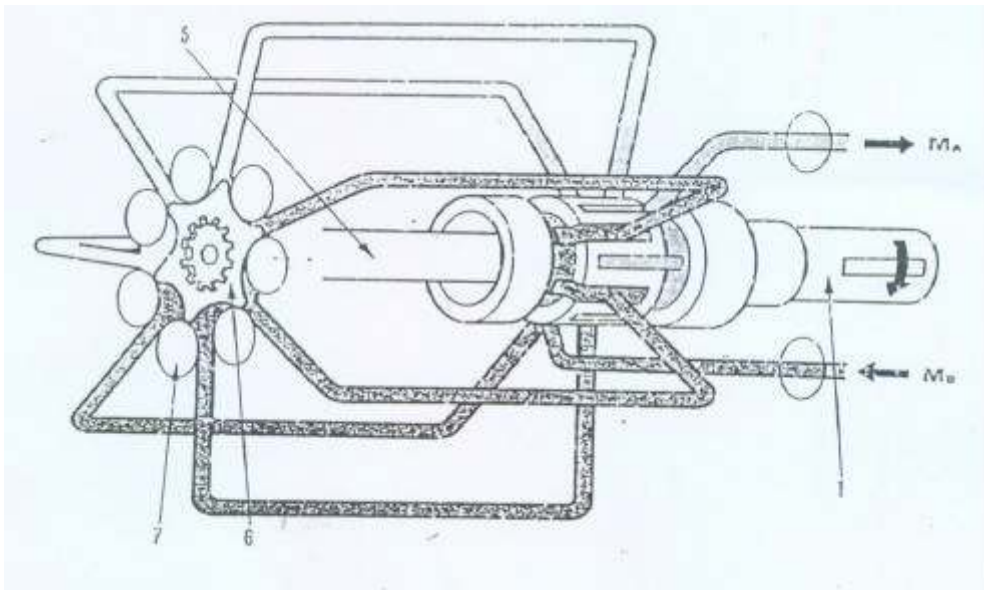
Gambar 4.163 Prinsip kerja orbit motor.
