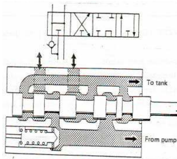
Gambar 4.128 ( d ). Katup pengontrol posisi float.
