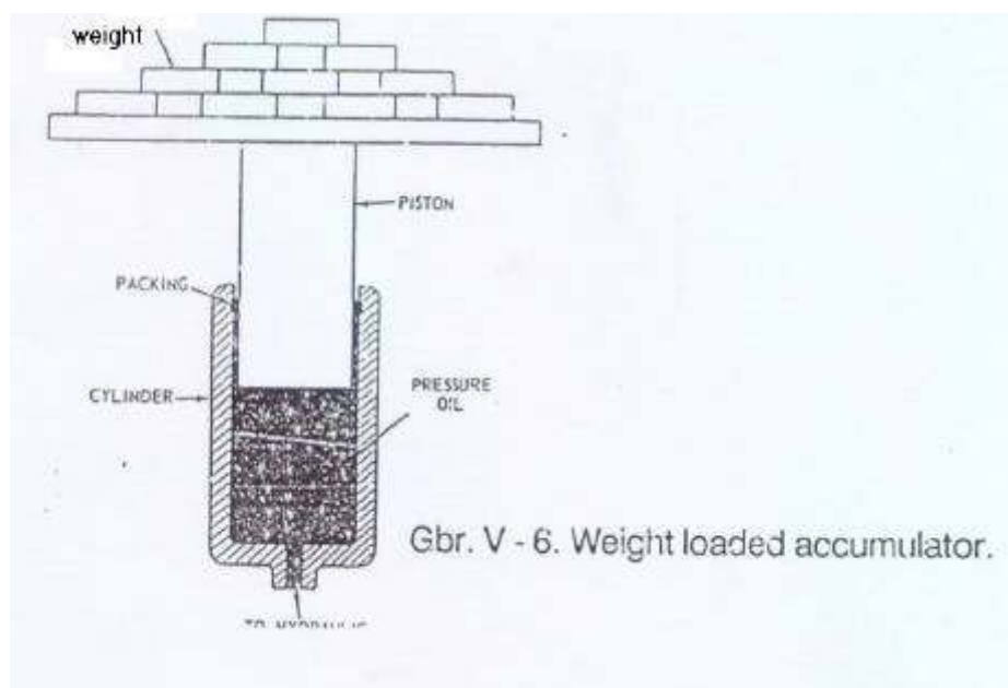
Gambar 4.169 Akumulator dengan beban pemberat
