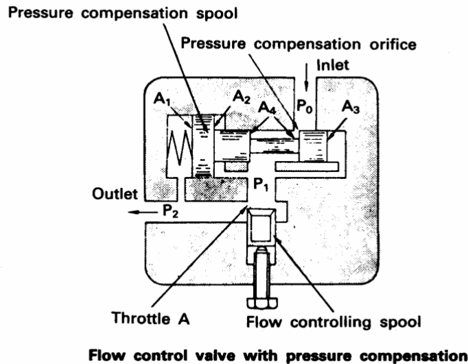
Gambar 4.82 Katup control aliran dengan kompensasi tekanan
