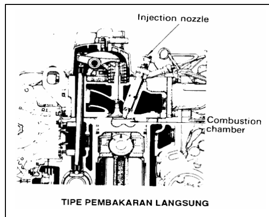
Gambar 4.17. Konstruksi Silinder Head Pembakaran Langsung
