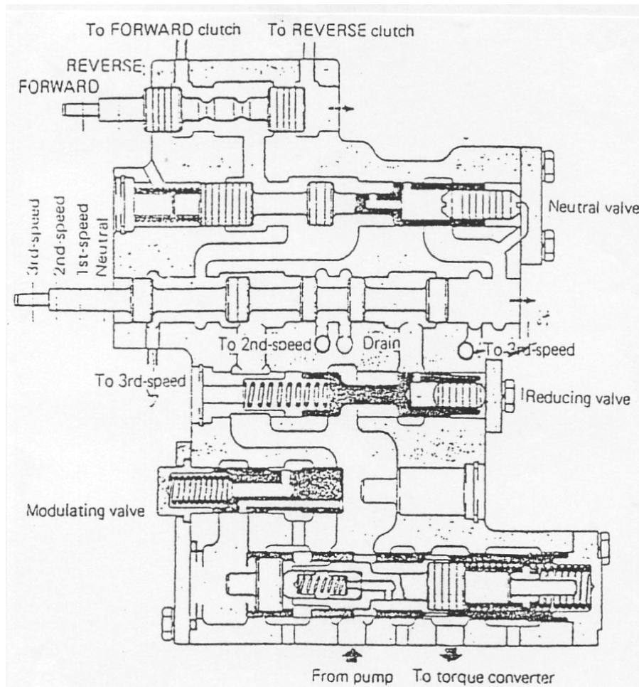
Gambar 4.212 contoh konstruksi Control Valve pada alat berat
