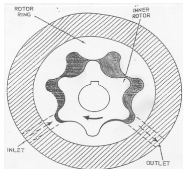
Gambar 4.69 Internal Gear Pump atau Pompa Trochoid
