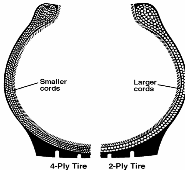
Gambar 4.143 Lapisan pada ban
