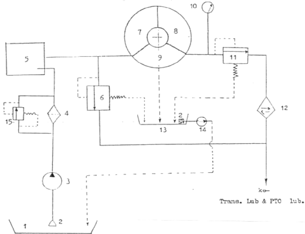
Gambar 4.187 Rangkaian hidrolik Torque Converter
