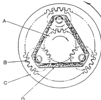
Gambar 4.200 Carrier ditahan
