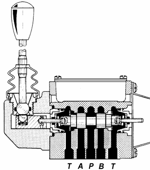
Gambar 4.86 Aktuator manual
