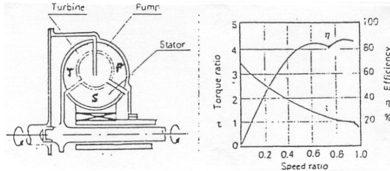
Gambar 4.180 Konstruksi dan grafik karakteristik Double Phase
