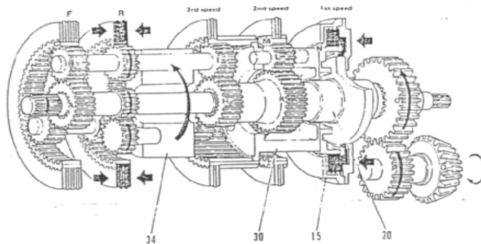
Gambar 4.208 Mundur Kecepatan 1
