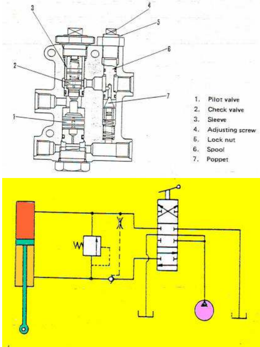
Gambar 4.131 (a) dan (b) Konstruksi dan simbol pilot check valve
