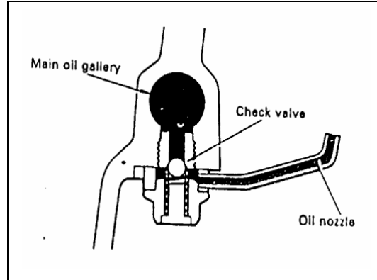
Gambar 4.37. Nosel Oli
