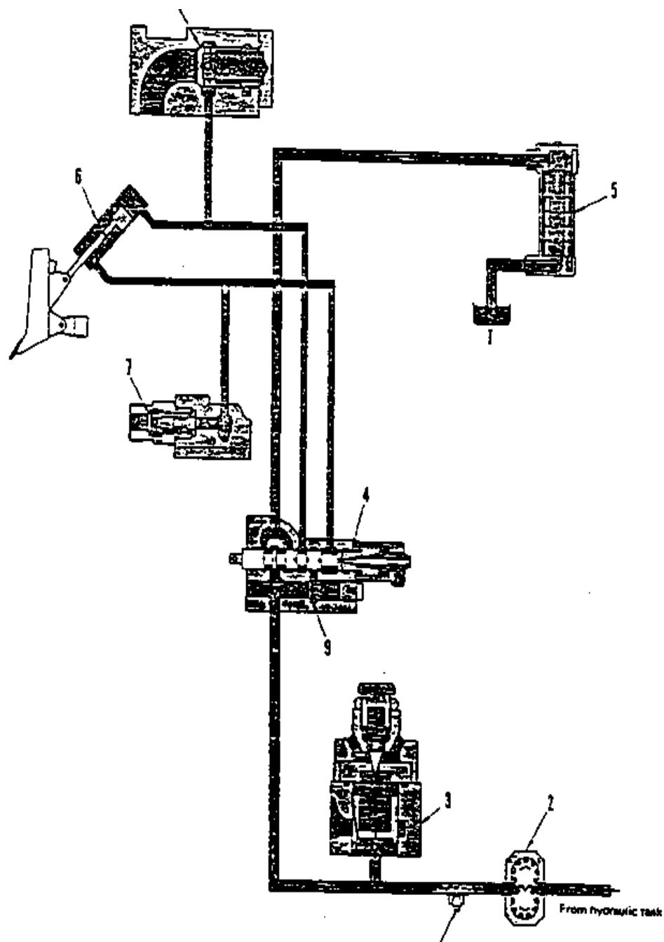
Gambar 4.144 Sistem kontrol Hidrolik pada Angledozer with Ripper (2 silinder) pada posisi netral
