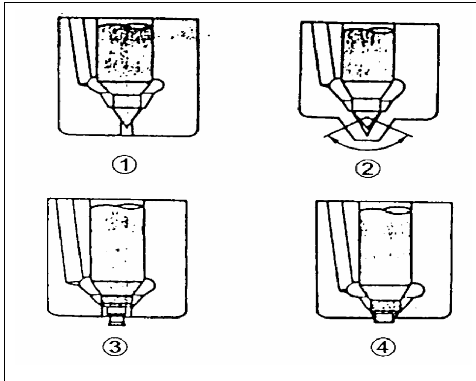
Gambar 4.47. Klasifikas Berdasarkan Penyemprotan
