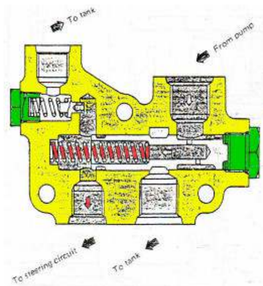
Gambar 4.117 Prinsip kerja flow divider (sebelum)
