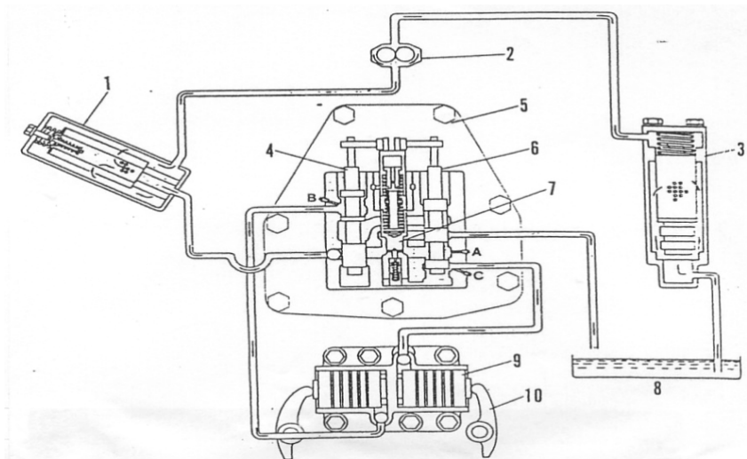
Gambar 4.120 Sirkuit oli untuk ke booster steering clutch
