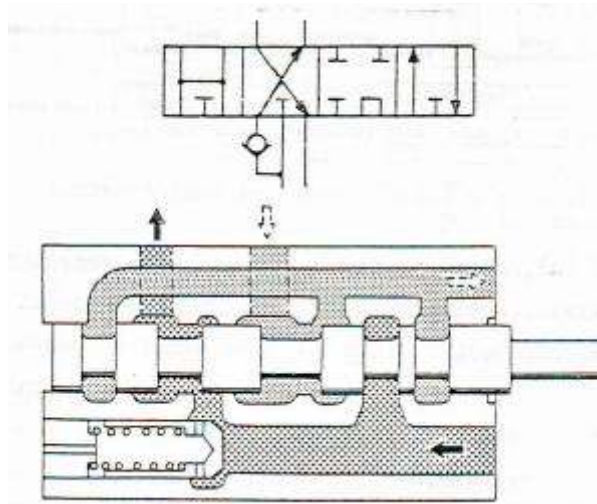
Gambar 4.128 ( c ). Katup pengontrol posisi lower
