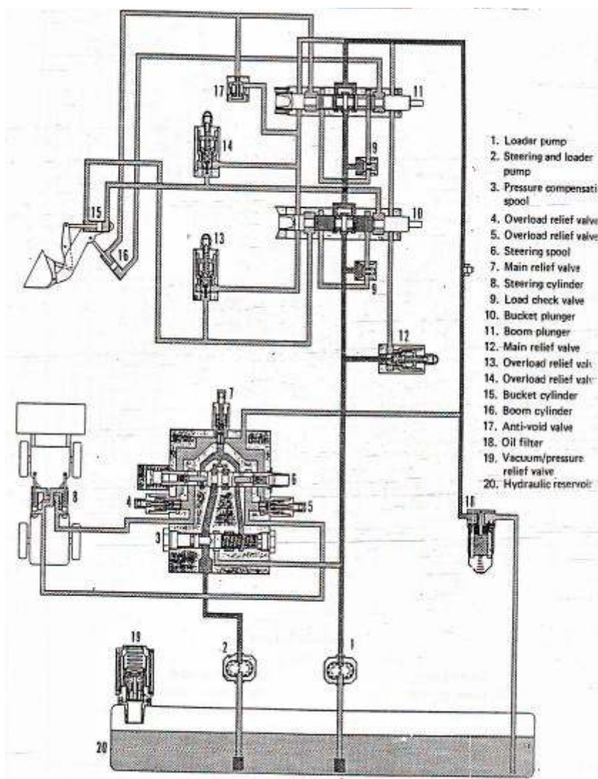
Gambar 4.122 (b) Skema hidrolis Wheel Loader W90-3
