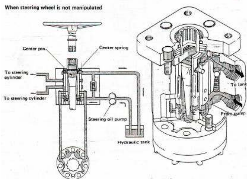
Gambar 4.132 (a) Konstruksi orbitroll valve
