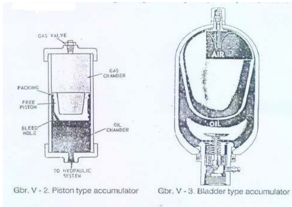
Gambar 4.167 Akumulator type piston dan bladder
