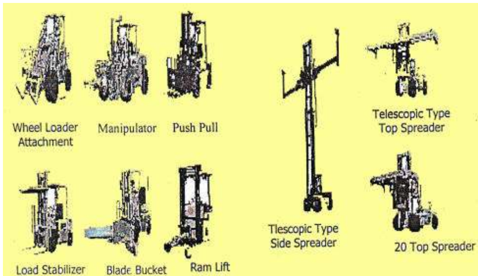
Gambar 5.36 Perlengkapan Forklift (2)
