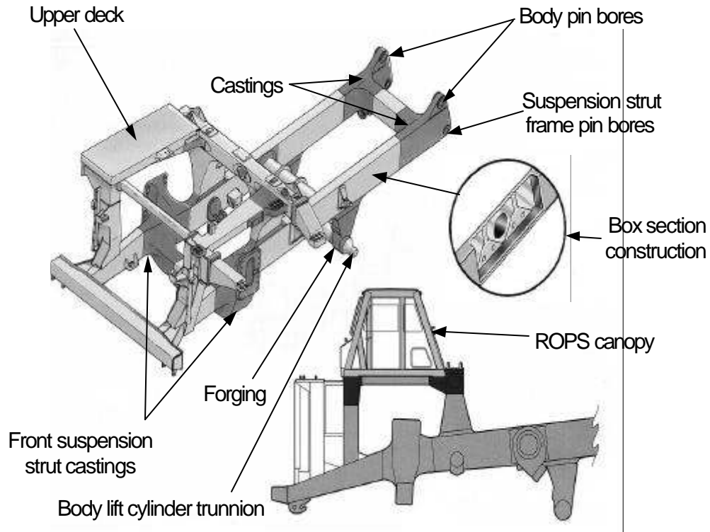
Gambar 4.154 Frame truk
