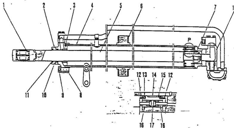
Gambar 4.140. Blade lift cylinder pada Bulldozer
