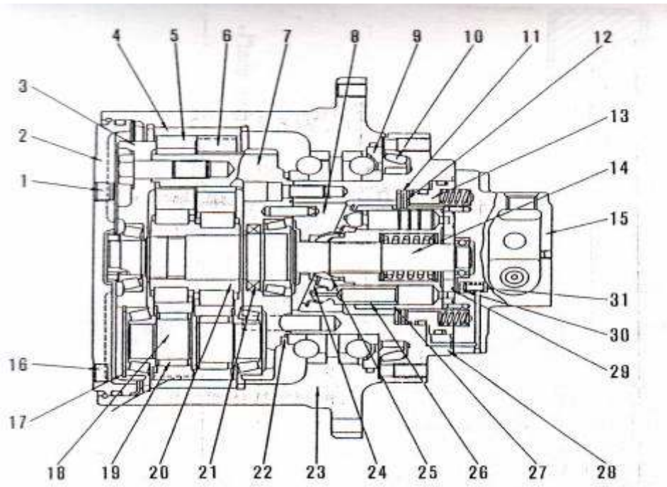
Gambar 4.160 Motor hidrolik tipe piston (swashplate)
