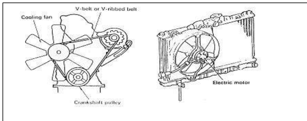
Gambar 4.27. Konstruksi Penggerak Kipas
