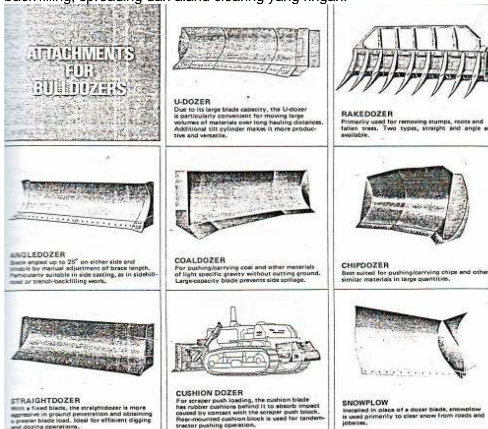
Gambar 5.24Perlengkapan bulldozer (1)
