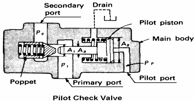
Gambar 4.97 Katup check dengan pemandu
