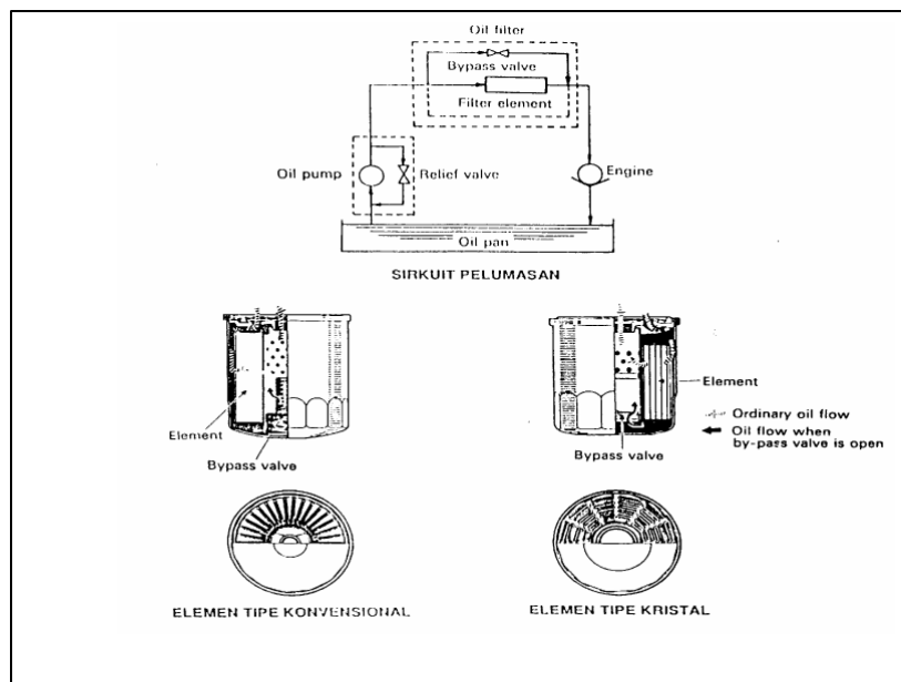
Gambar 4.34. Konstruksi Filter Oli
