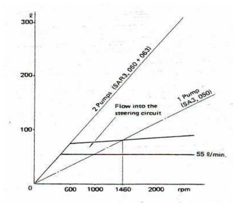
Gambar 4. 121 Karakteristik aliran pada demand valve
