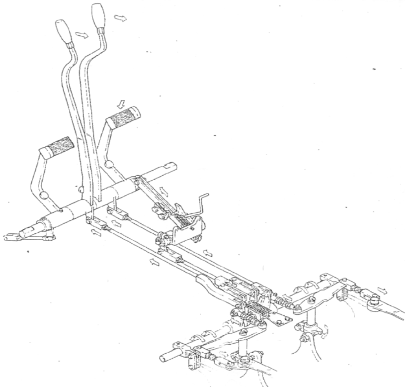
Gambar 4.117 Konstruksi Steering Linkage
