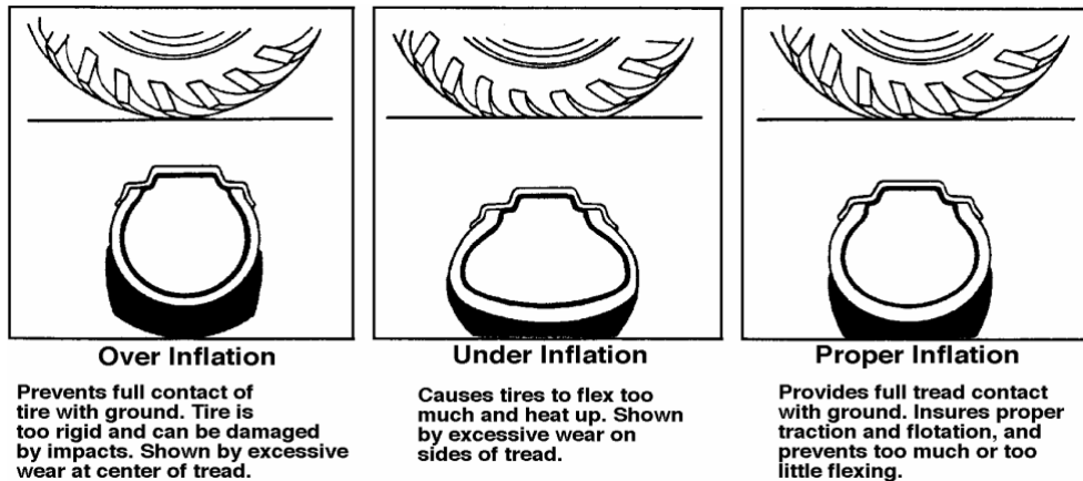
Gambar 4.146 Pemompaan pada ban
