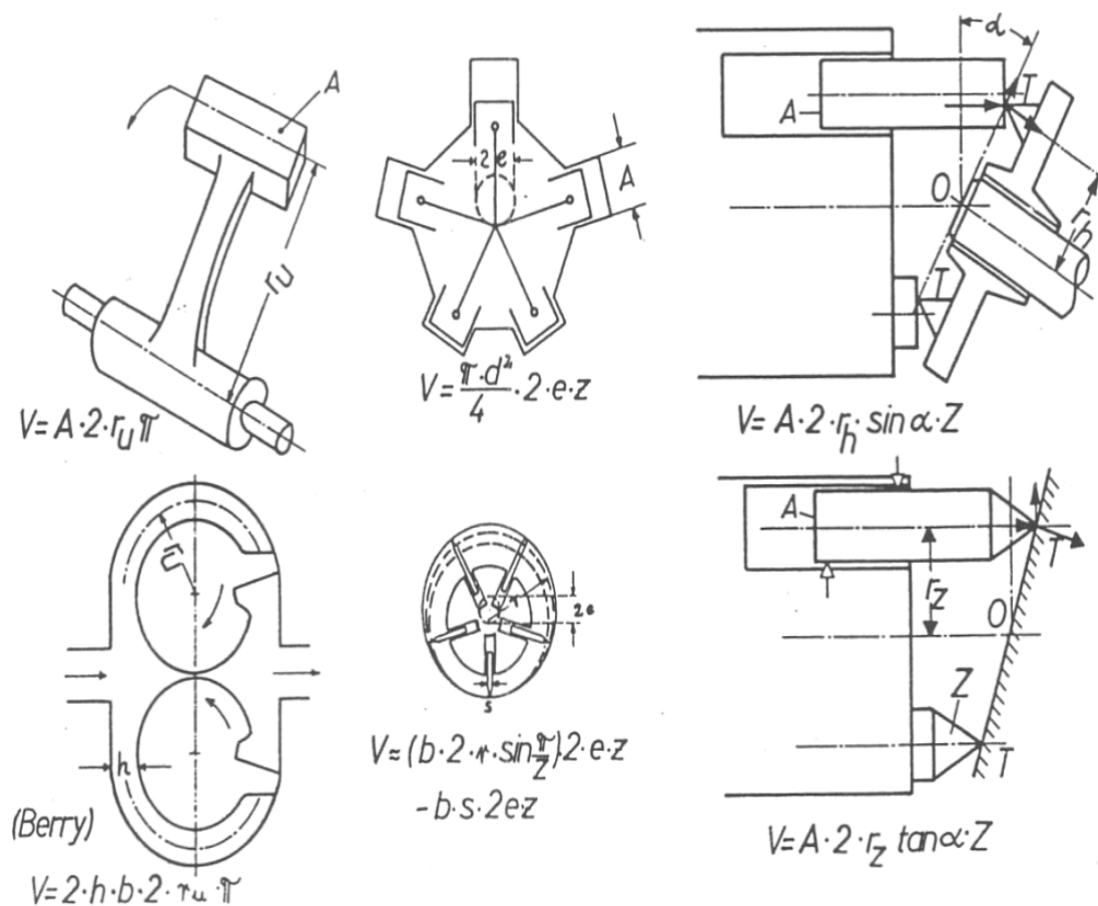
Gambar 4.63 Pembentukan volume pada mesin hidrostatis
