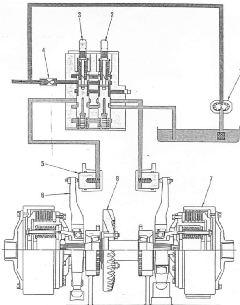
Gambar 4.122 Konstruksi dan sirkuit sistem semi hidrolik untuk D3 1-17
