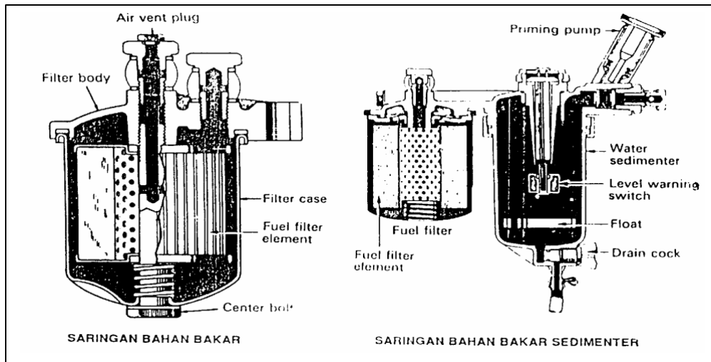
Gambar 4.41. Saringan Bahan Bakar dan Sedimenter
