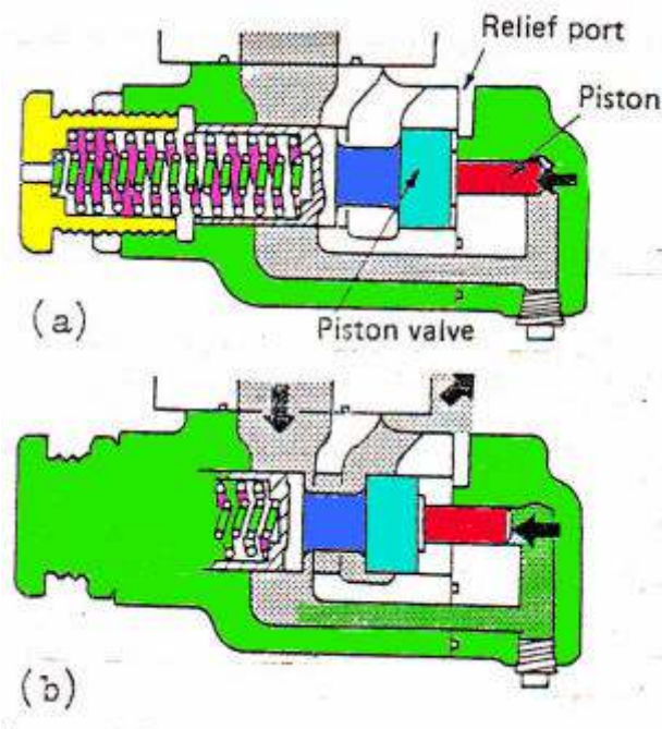
Gambar. 4.108 Prinsip kerja tipe piston
