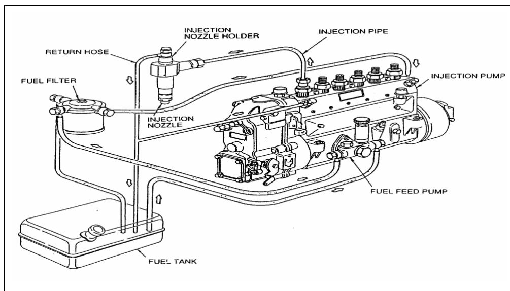
Gambar 4.39. Proses Aliran Bahan Bakar Pada Motor Diesel
