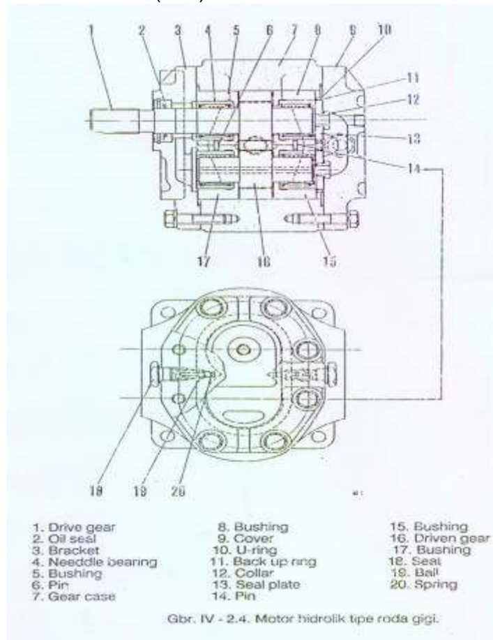
Gambar 4.154 Motor hidrolik type roda gigi luar
