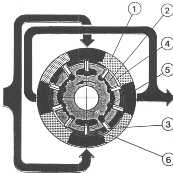
Gambar 4.67 Konstruksi pompa sudu
