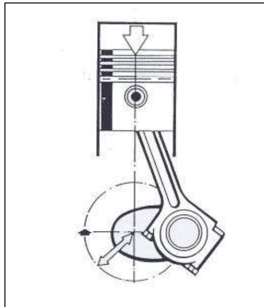
Gambar 4.50. Momen Pada Poros Engkol
