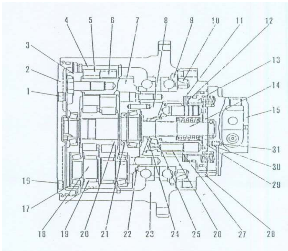
Gambar 4.161 Motor hidrolik tipe piston (bent)
