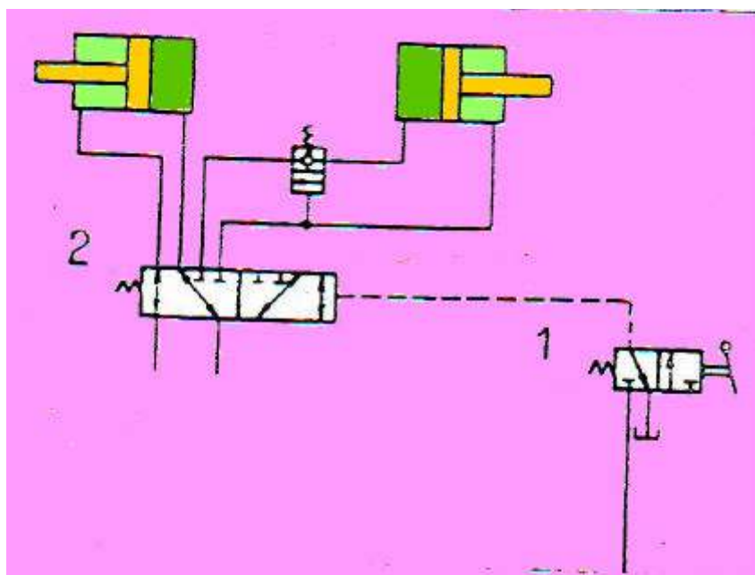
Gambar 4.133 (a) dan (b) Prinsip kerja dan Simbol actuator dan ripper selector valve
