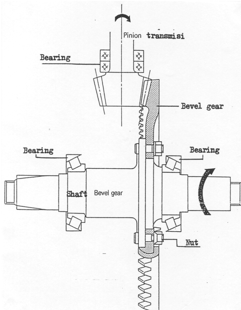
Gambar 4.141 Skema arah putaran dari transmisi ke bevel gear
