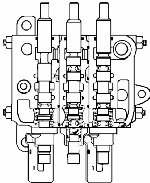
Gambar 4.92 Katup kontrol arah ganda/paralel
