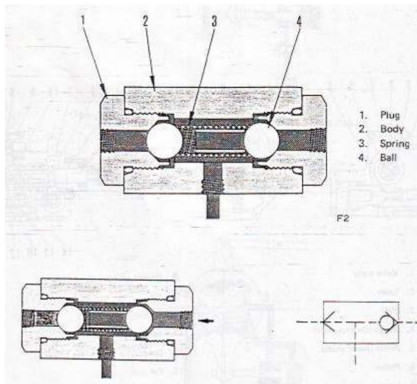
Gambar 4.136. Konstruksi, simbol dan prinsip kerja shuttle valve.
