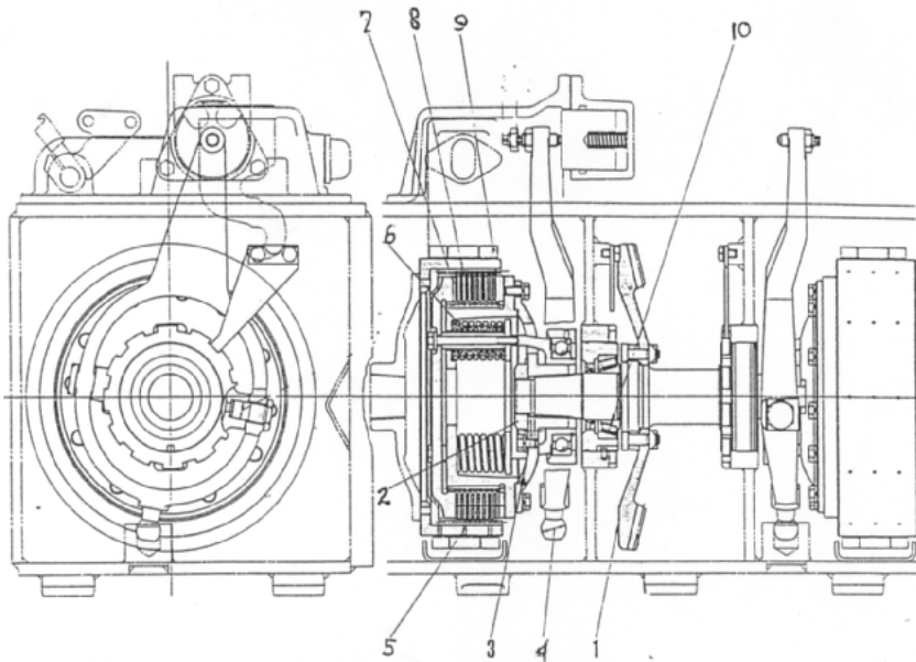
Gambar 4.121 Konstruksi lengkap sistem semi hidrolis
