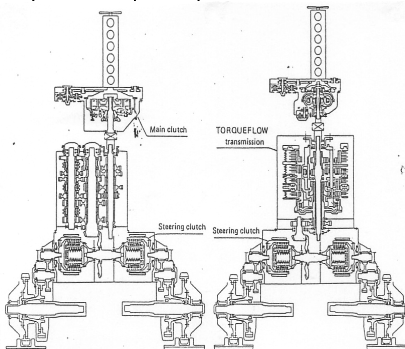
Gambar 4.114 Konstruksi Bulldozer/Shovel dari mesin-roda crawler
