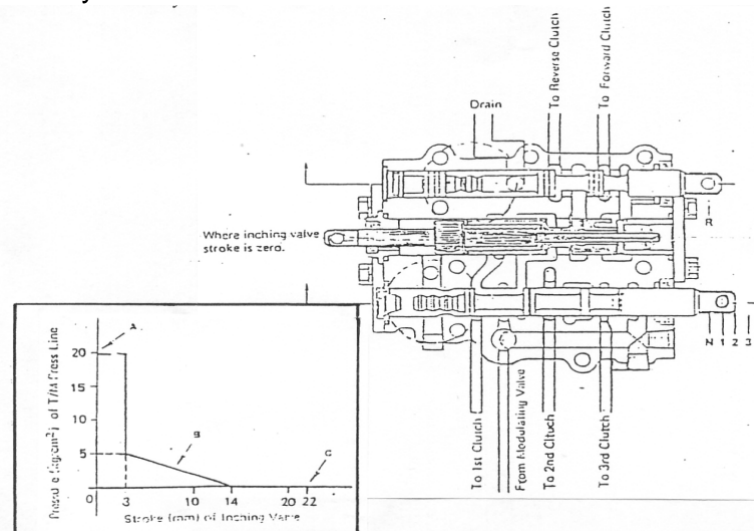
Gambar 4.113 Konstruksi Inching Valve dan karakteristiknya
