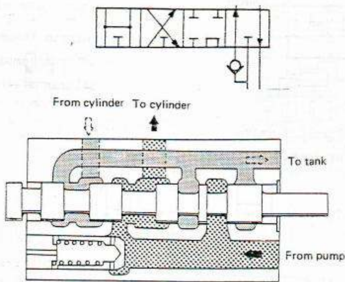
Gambar 4.128 (b) Katup pengontrol posisi raise
