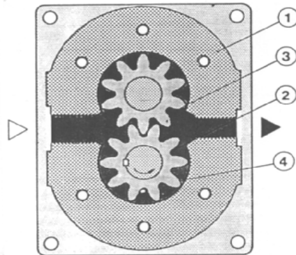
Gambar 4.65 Pompa roda gigi dengan roda gigi luar
