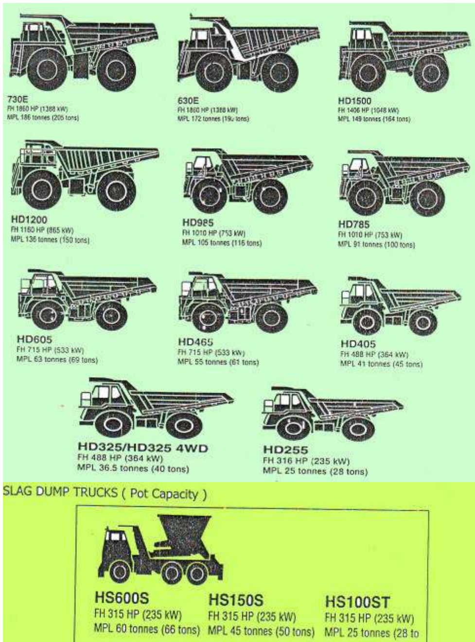
Gambar 5.37 Produk Dumptruck Komatsu
