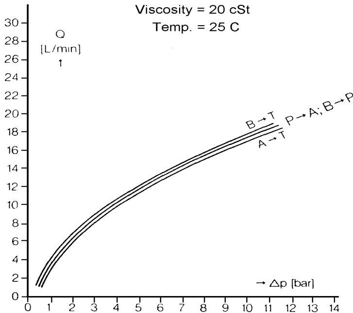
Gambar 4.83 Karakteristik Katup 4/3 Contoh dan kalkulasi diperlihatkan pada halaman berikut
