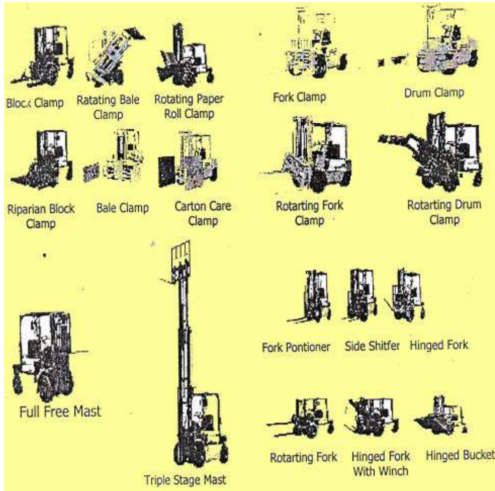
Gambar 5.35 Perlengkapan Forklift (1)
