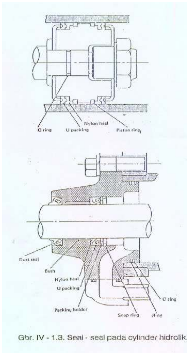
Gambar 4.147 Seal-seal pada silinder hidrolis
