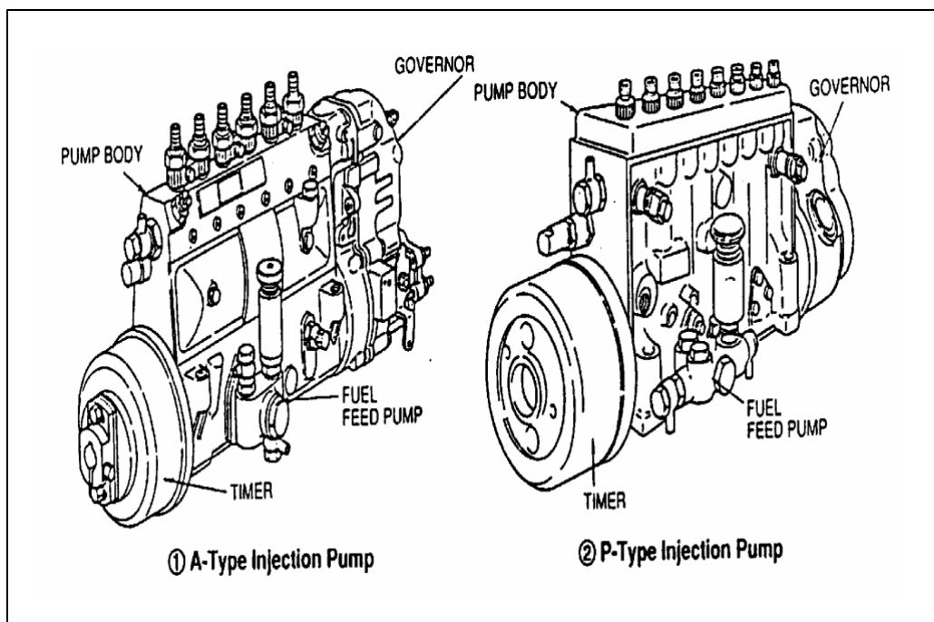
Gambar 4.45. Pompa Injeksi Tipe In-line
