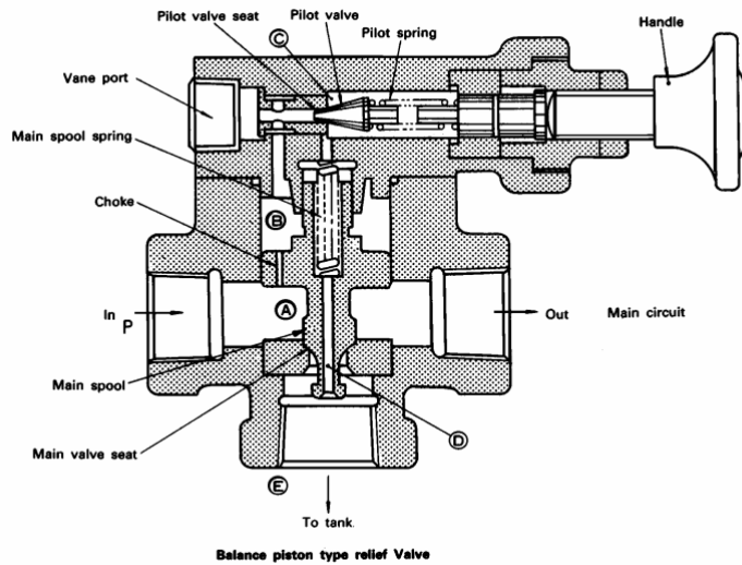
Gambar 4.78 Katup relief
