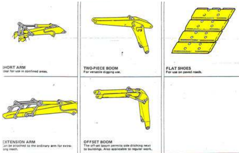
Gambar 5.9 Berbagai perlengkapan pada Excavator (3)
