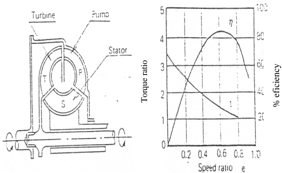
Gambar 4.177 Konstruksi dan grafik karakteristik Single Phase
