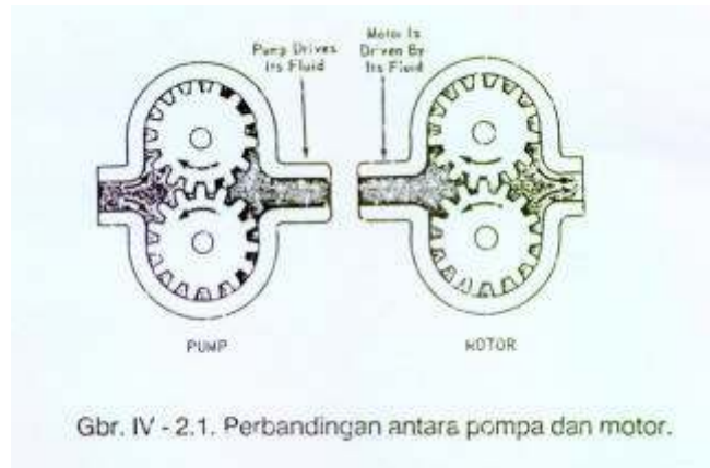
Gambar 4.152 Perbandingan pompa dan motor hidrolis
