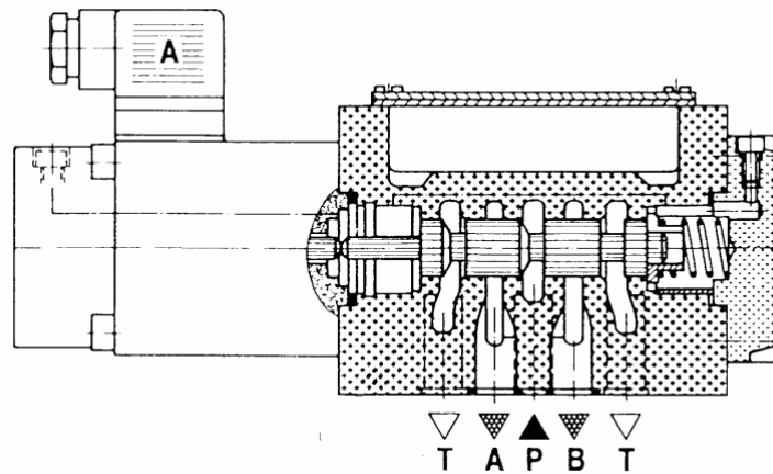
Gambar 4.87 Katup dua posisi yang dioperasikan oleh solenoid tunggal
