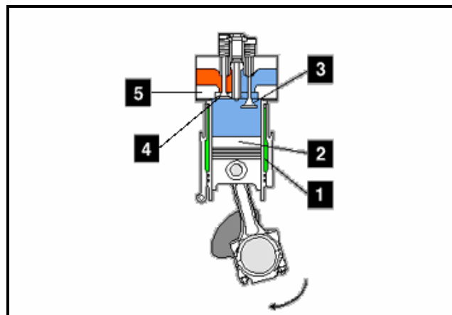
Gambar 4.6 Komponen Engine Pembentuk Ruang Bakar
