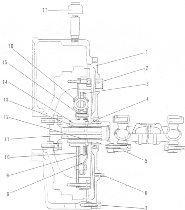
Gambar 4.175. Konstruksi Damper dan nama-nama bagian Damper
