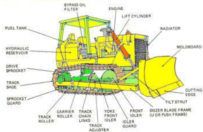
Gambar 5.17 Nama bagian Track-type tractor
