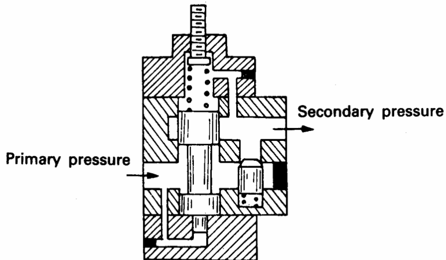
Gambar 4.81 Katup penyeimbang
