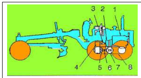
Gambar 5.13 Nama Komponen Motor Grader
