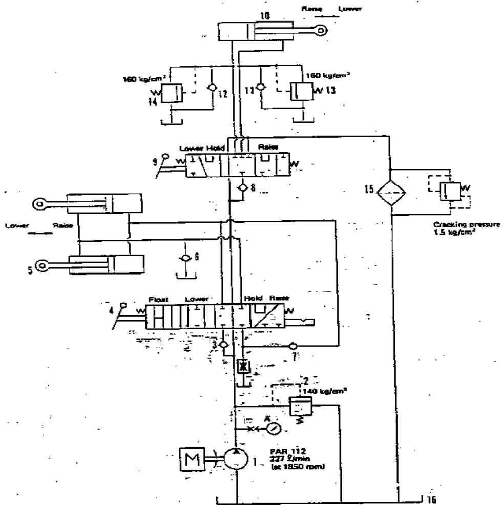
Gambar 4.143 Sirkuit Sistem Hidrolik pada Angledozer with Ripper (2 silinder)
