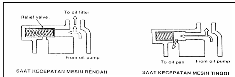
Gambar 4.33. Pengaturan Oleh Relief Valve
