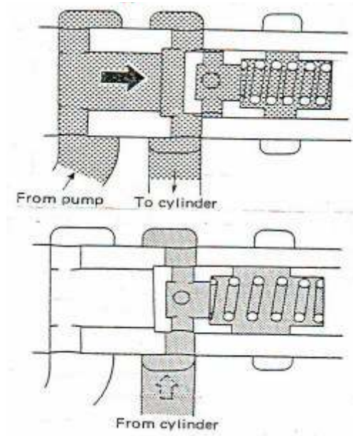
Gambar 4. 129 Katup satu arah (check valve)
