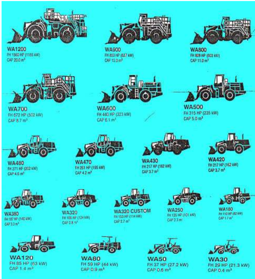
Gambar 5.44 Produk Wheel Loader Komatsu (1)
