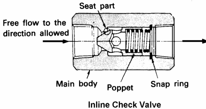
Gambar 4.96 Katup check
