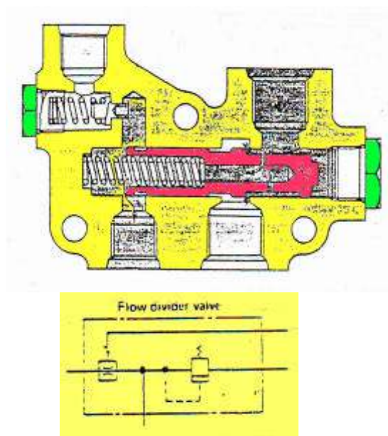
Gambar 4.118 Flow devider (bekerja) & simbolnya
