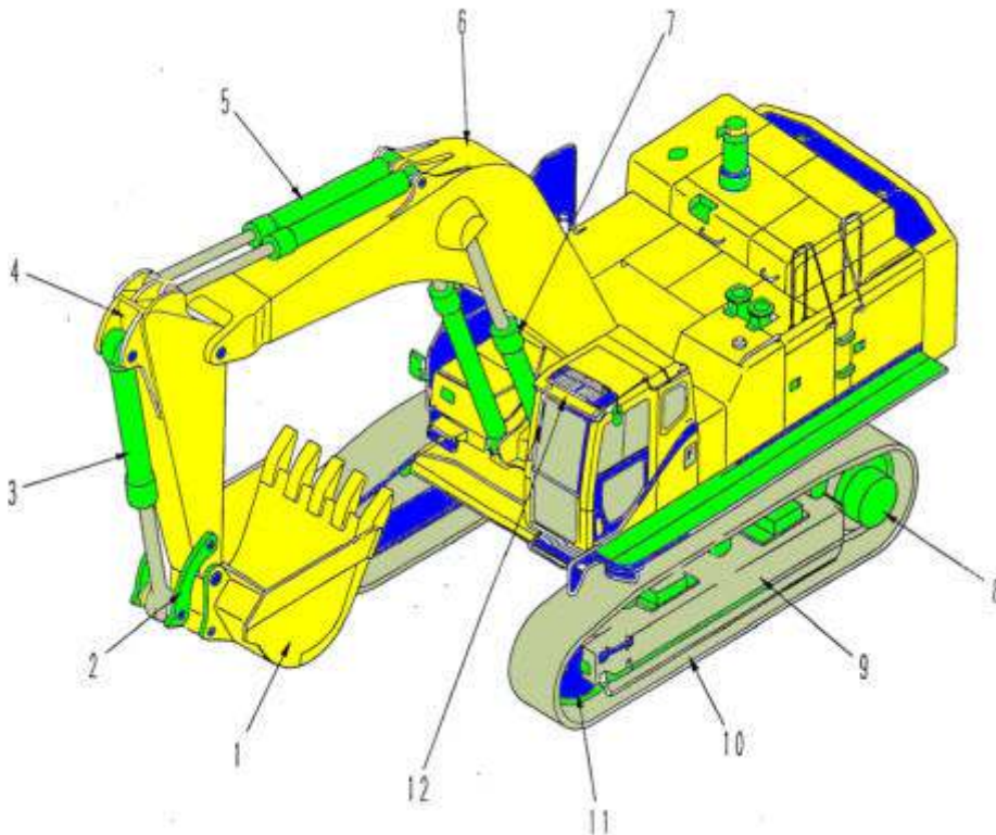
Gambar 5.4 Nama bagian Excavator
