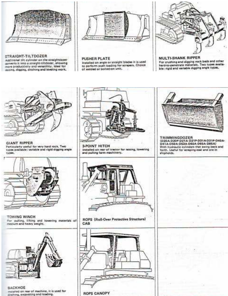
Gambar 5.25 Perlengkapan Bulldozer (2)
