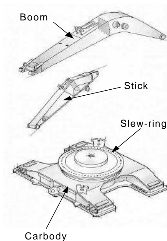
Gambar 156 Frame ekskavator
