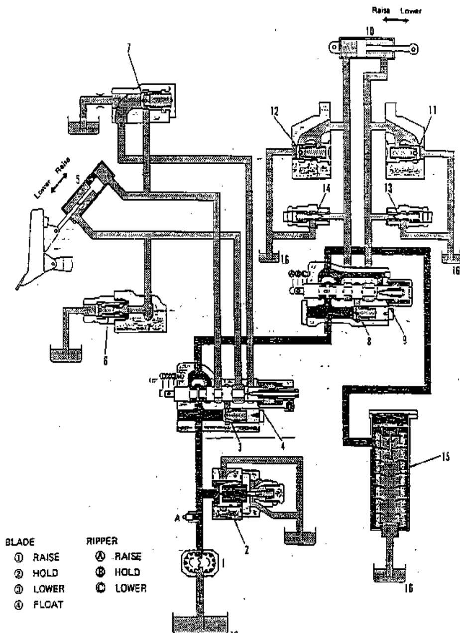
Gambar 4.142. Sistem kontrol Hidrolik pada Angledozer with Ripper (2 cyl)
