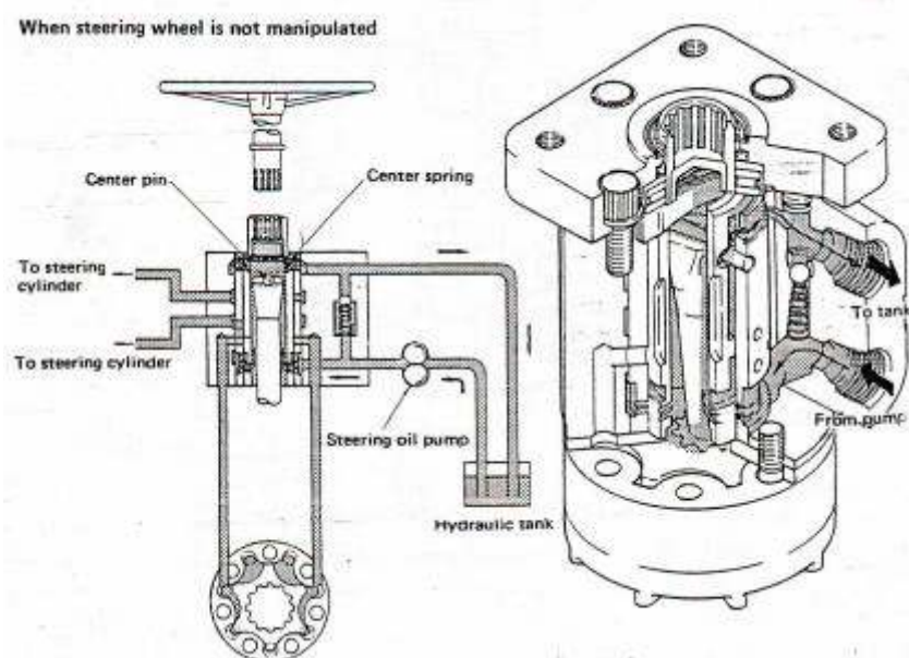
Gambar 4.132 (c) Prinsip kerja orbitrol valve sebagai directional control valve.
