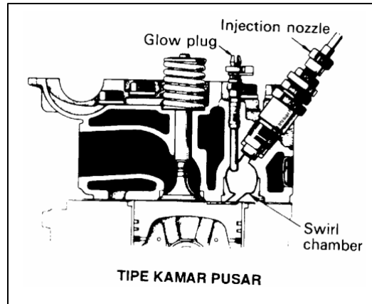
Gambar 4.16 Konstruksi Silinder Head Pemb. Tak Langsung
