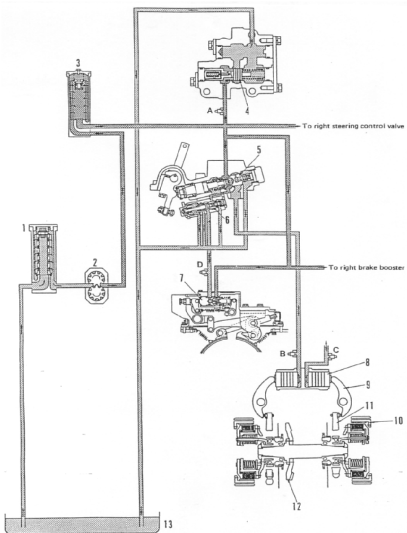
Gambar 4.123 Konstruksi dan sirkuit sistem semi hidrolik untuk D50,53-17
