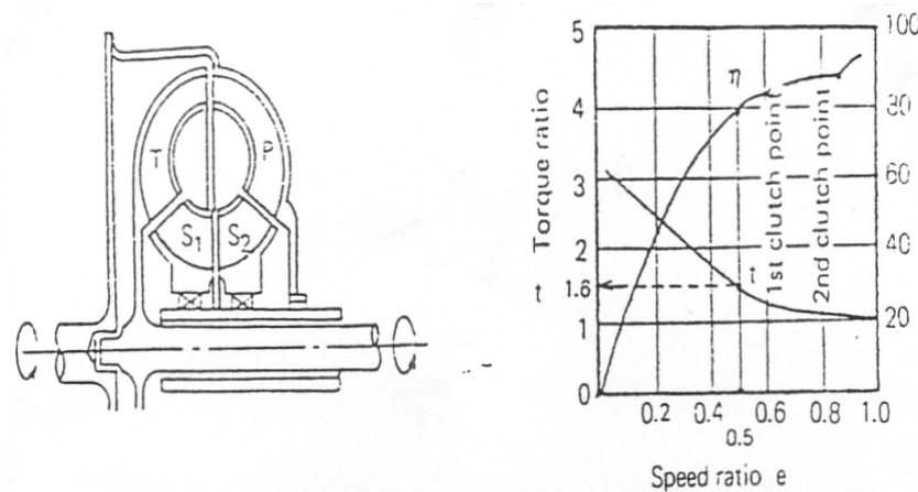
Gambar 4.181. Konstruksi dan grafik karakteristik Three Phase
