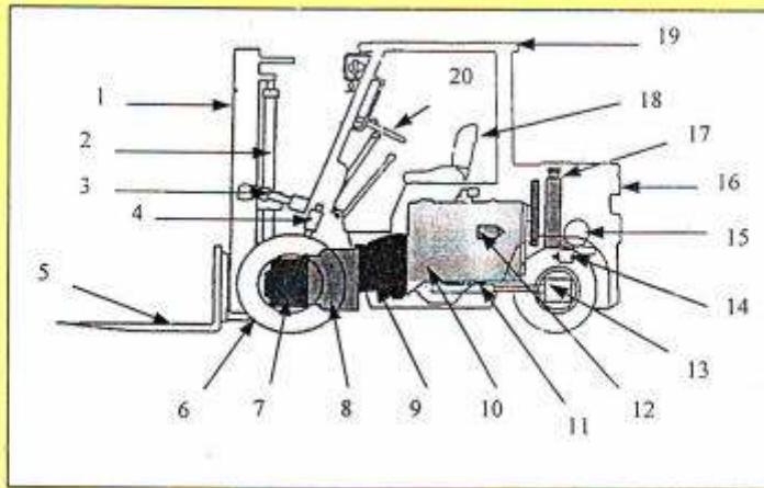
Gambar 5.31. Komponen Forklift
