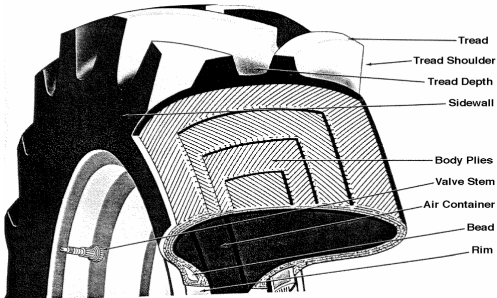
Gambar 4.142 Profil Ban
