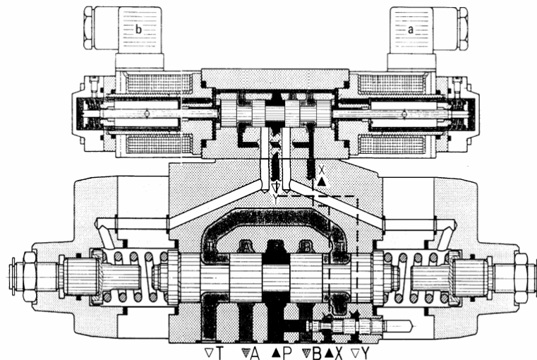
Port "X" adalah suplai pilot eksternal Port "Y" adalah aliran pembuangan pilot eksternal Gambar 4.90 Katup dua tingkat dengan pengontrolan solenoid
