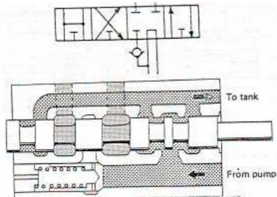
Gambar 4.128 (a). Katup pengontrol posisi netral.
