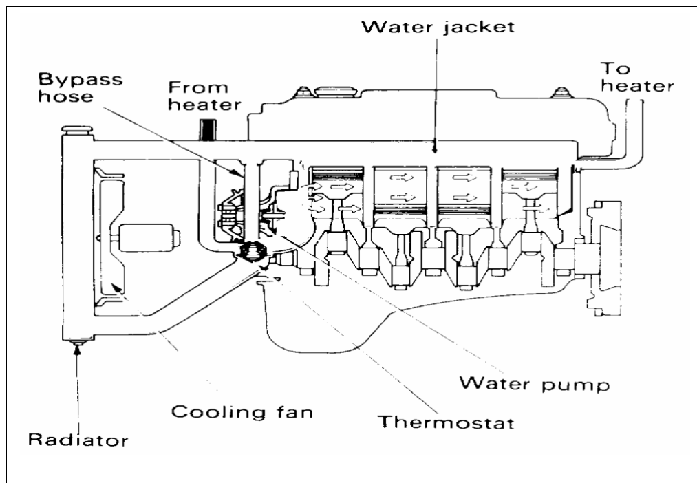
Gambar 4.18. Proses Pendinginan Saat Mesin Dingin
