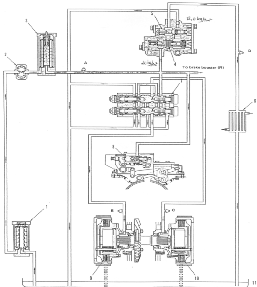
Gambar 4.127 Sirkuit steering Clutch D75s-3,5
