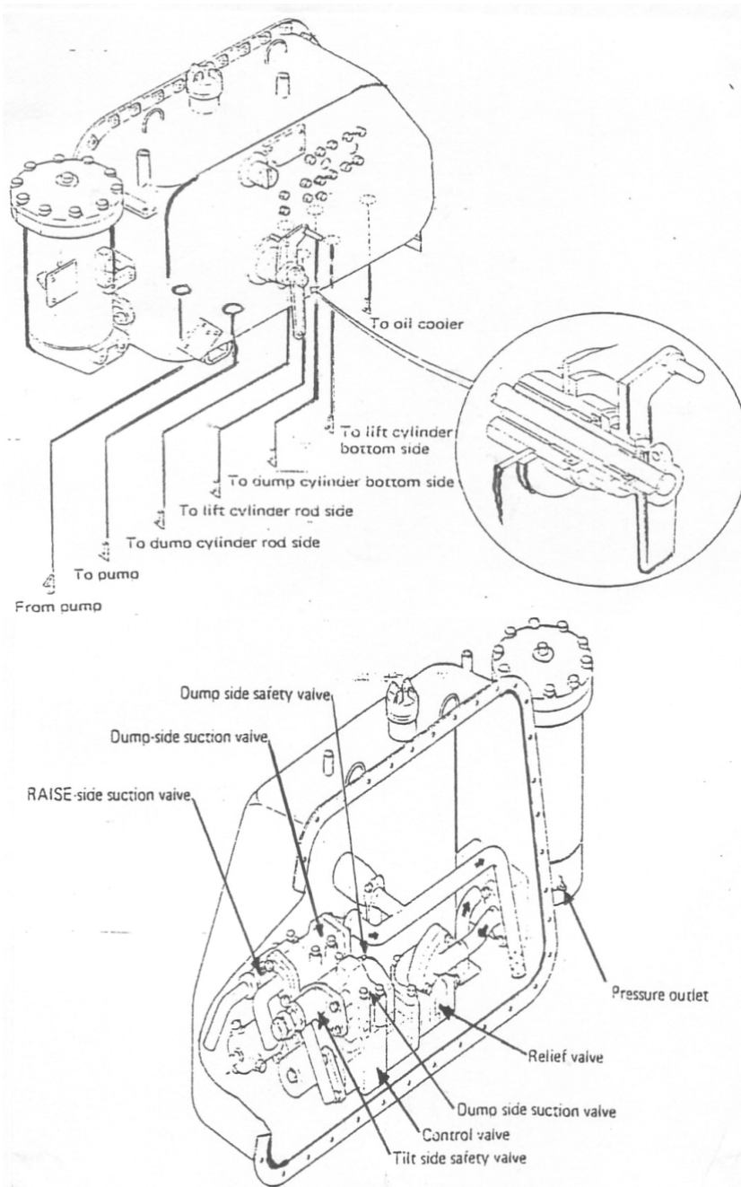
Gambar 4.52 Konstruksi Tangki hidrolis (3 dimensi)
