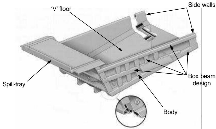
Gambar 4.155 Bed truk
