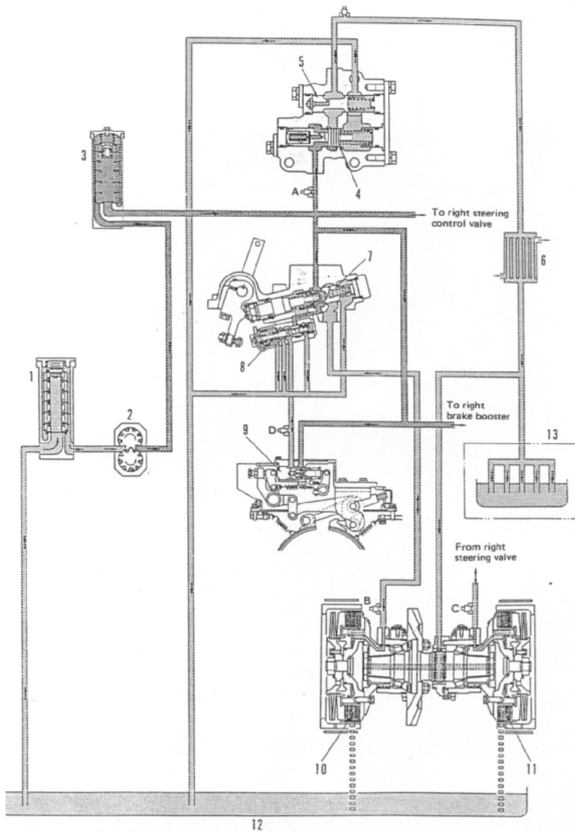
Gambar 4.125 Sirkuit steering clutch D60, 65-7,8
