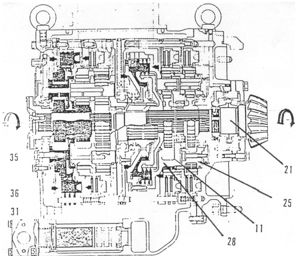
Gambar 4.209 Power Train kecepatan 1
